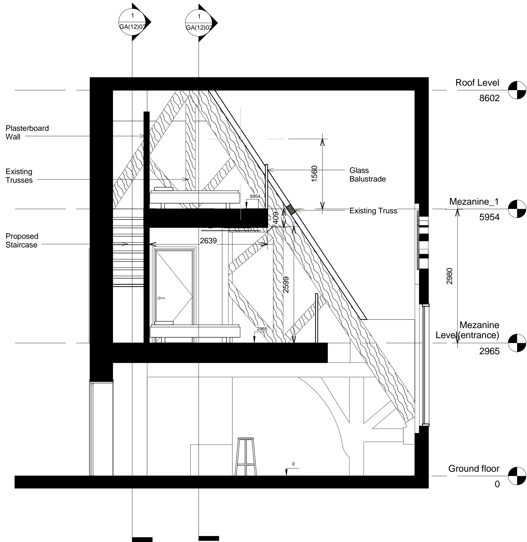
1 Section AA 1 : 50
