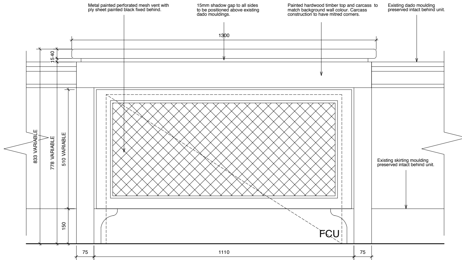
3 Front Elevation B Scale: 1:5
