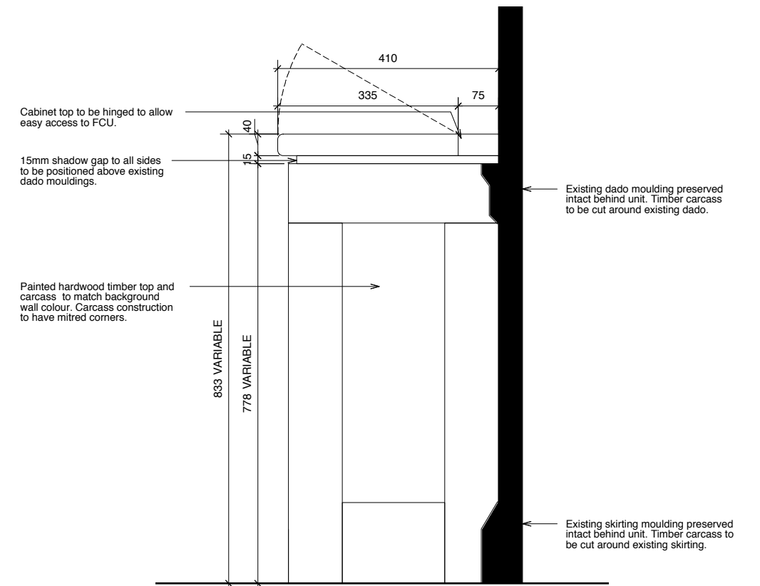
2 Section A Scale: 1:5
