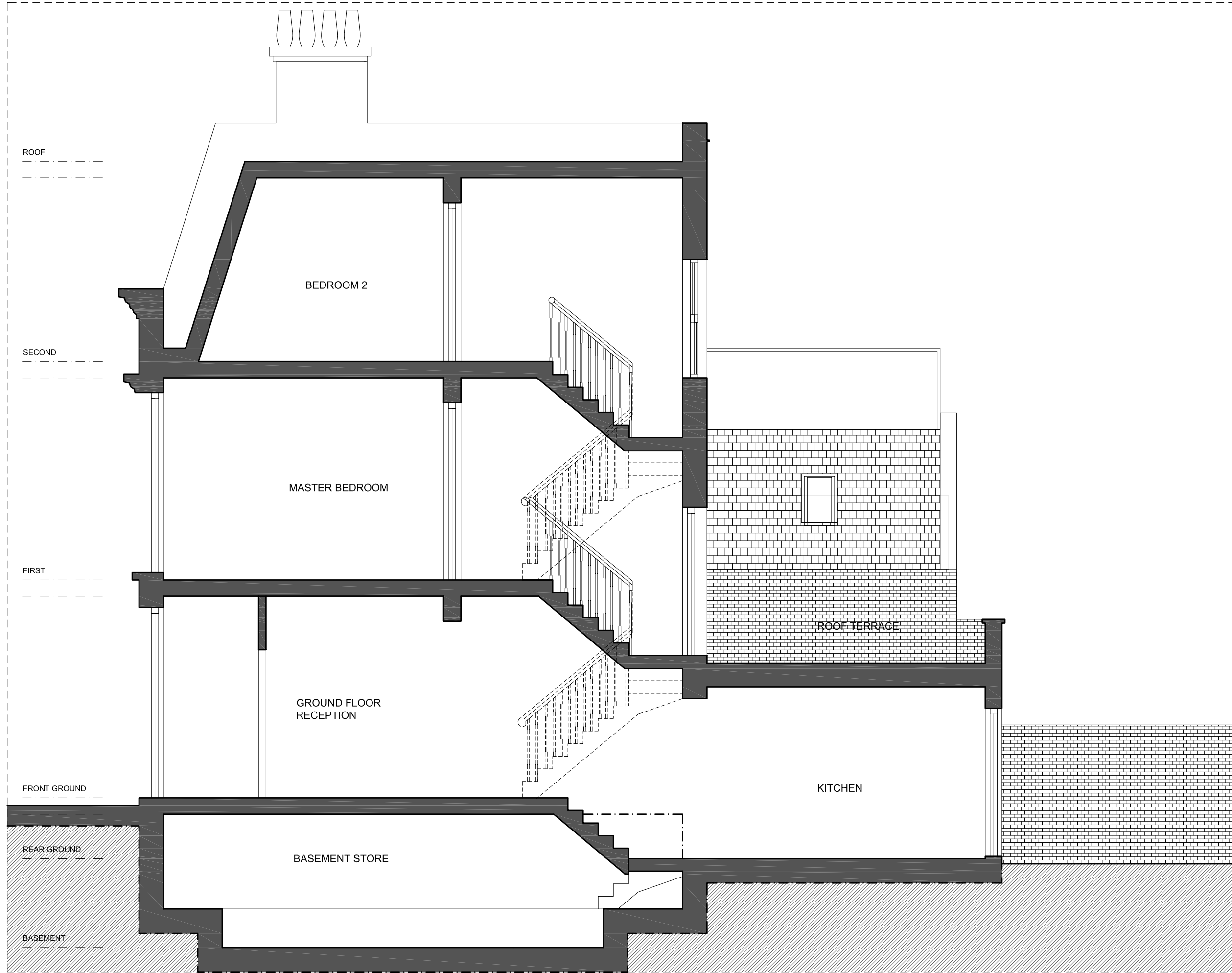
01 EXISTING SECTION A 1.50 @ A3
