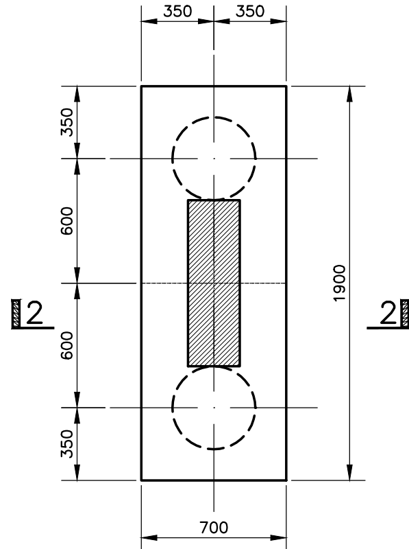
P02 Pile Cap Scale 1:25
