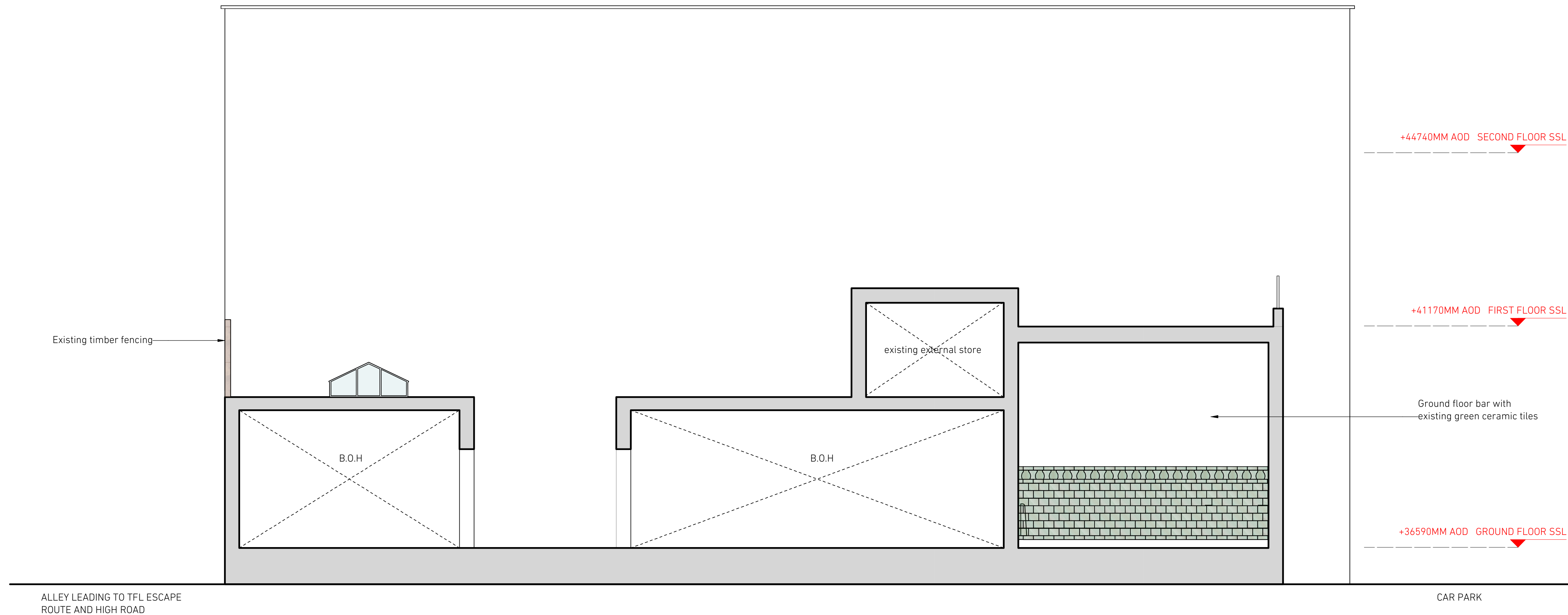
1 EXISTING SECTION G-G Scale: 1:50
