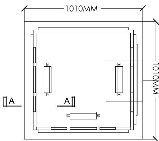
PLAN 1:20
