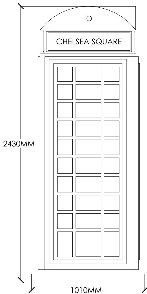
ELEVATION 1:20
