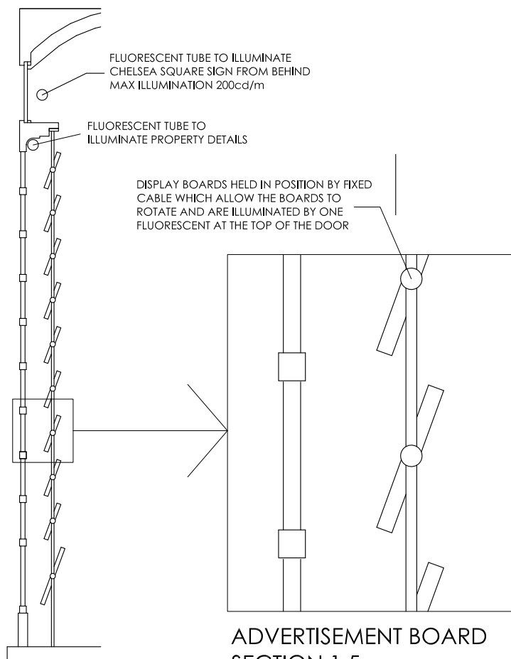
SECTION A-A 1:20
