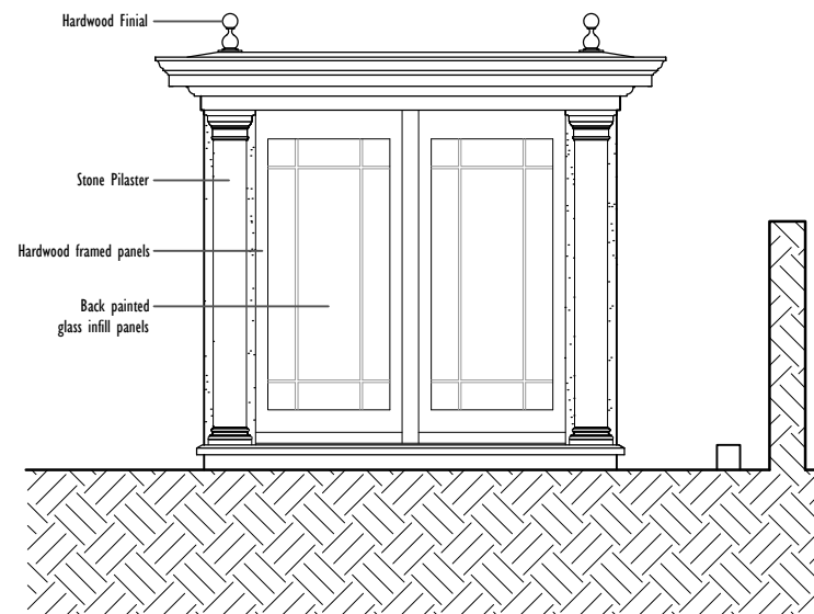
Elevation 1
