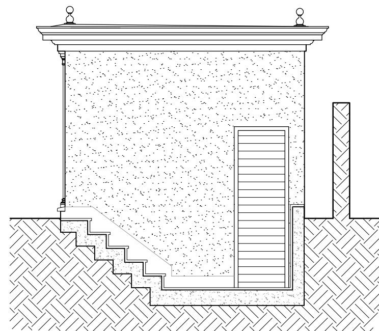
Elevation 2
