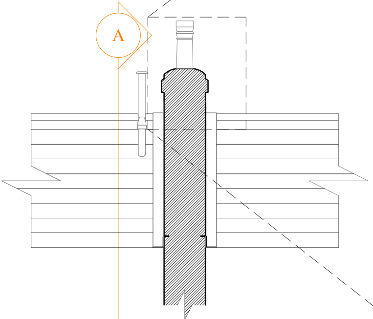
Section B~B 1:50
