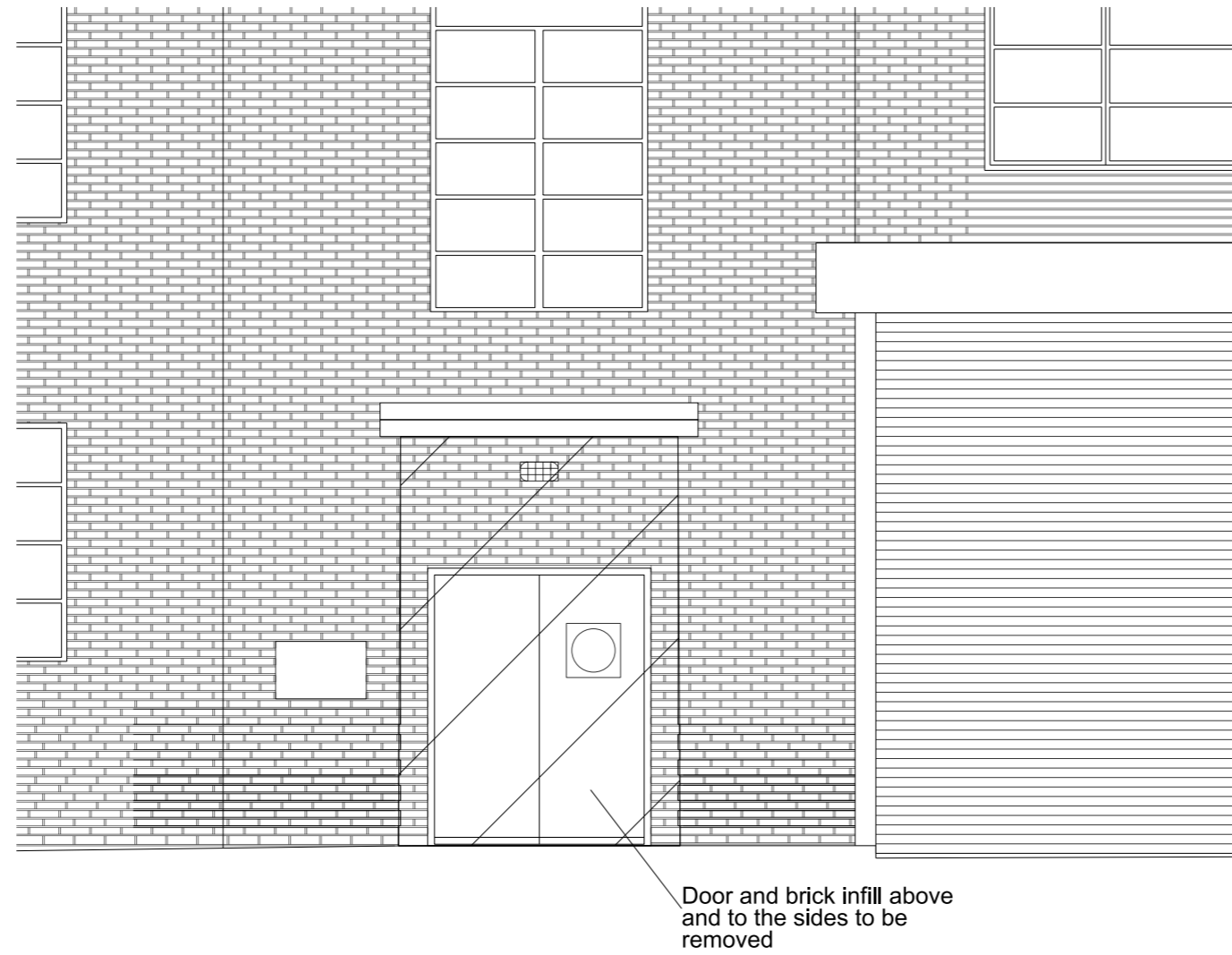
Elevation
