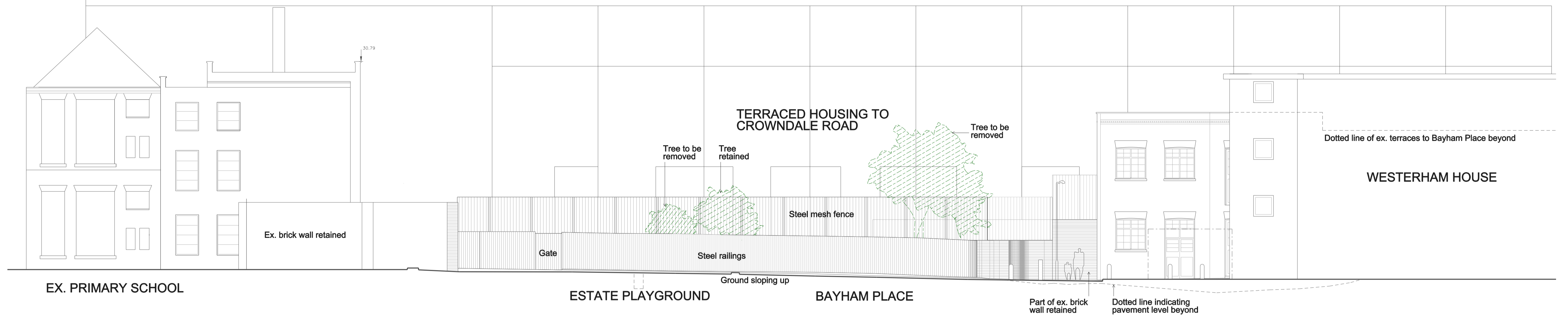
ELEV. 1
