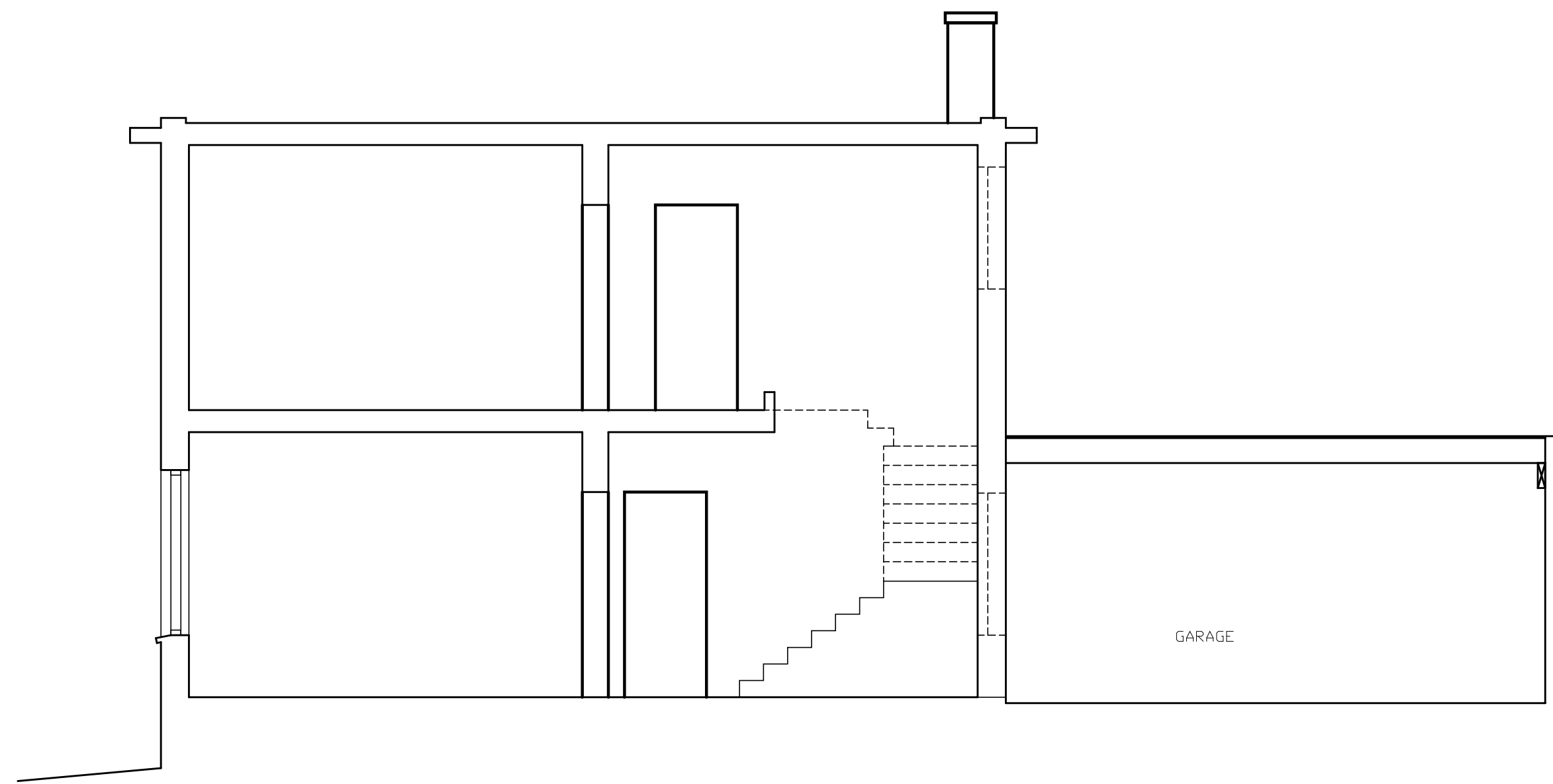
Section A-A
