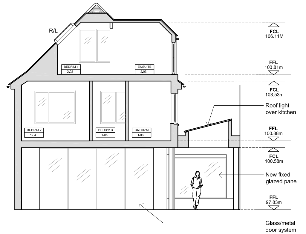
SECTION B - B 2 1:100 HIW-200
