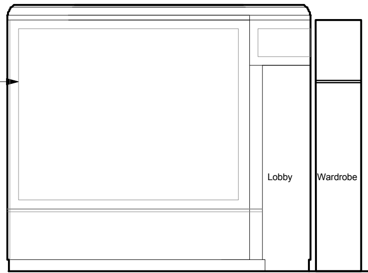
Elevation B
