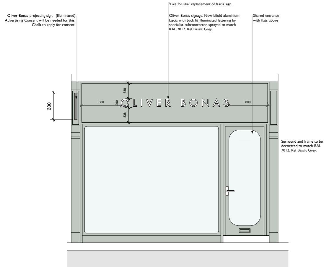
1 Elevation FF'
