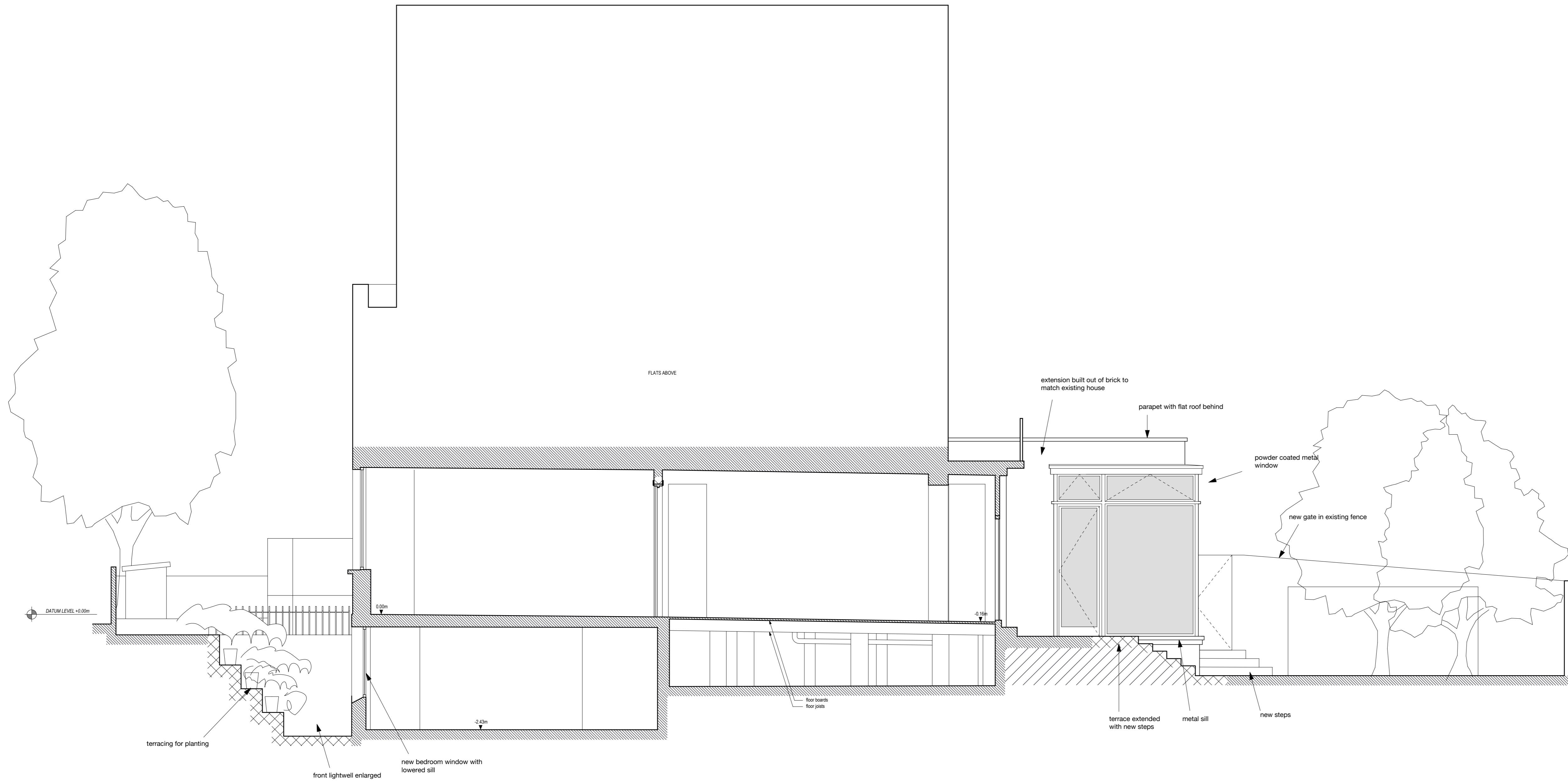
01_SECTION
