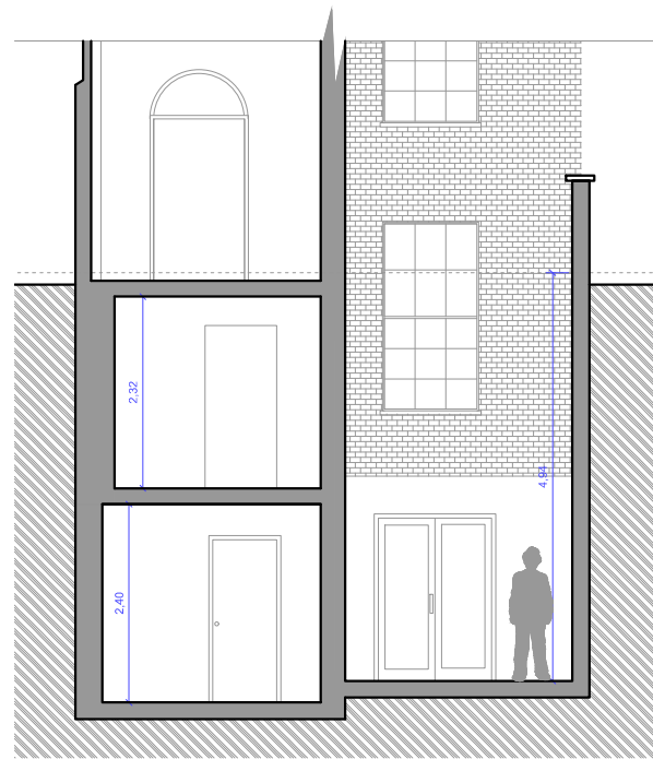
SECTION A-A' E: 1/100
