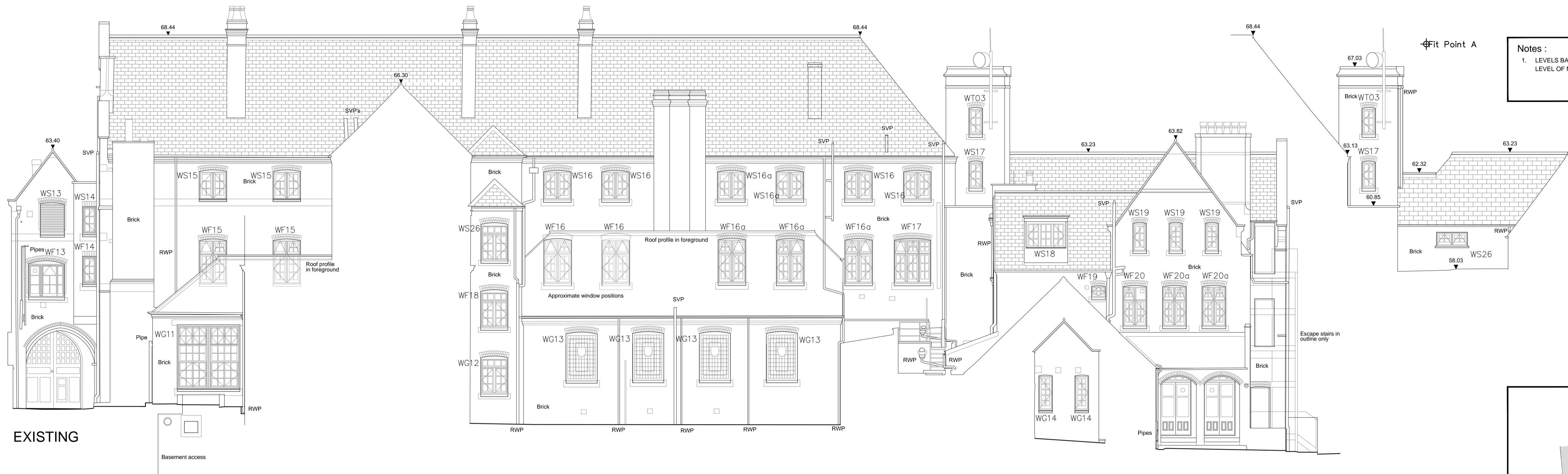
Elevation 4
