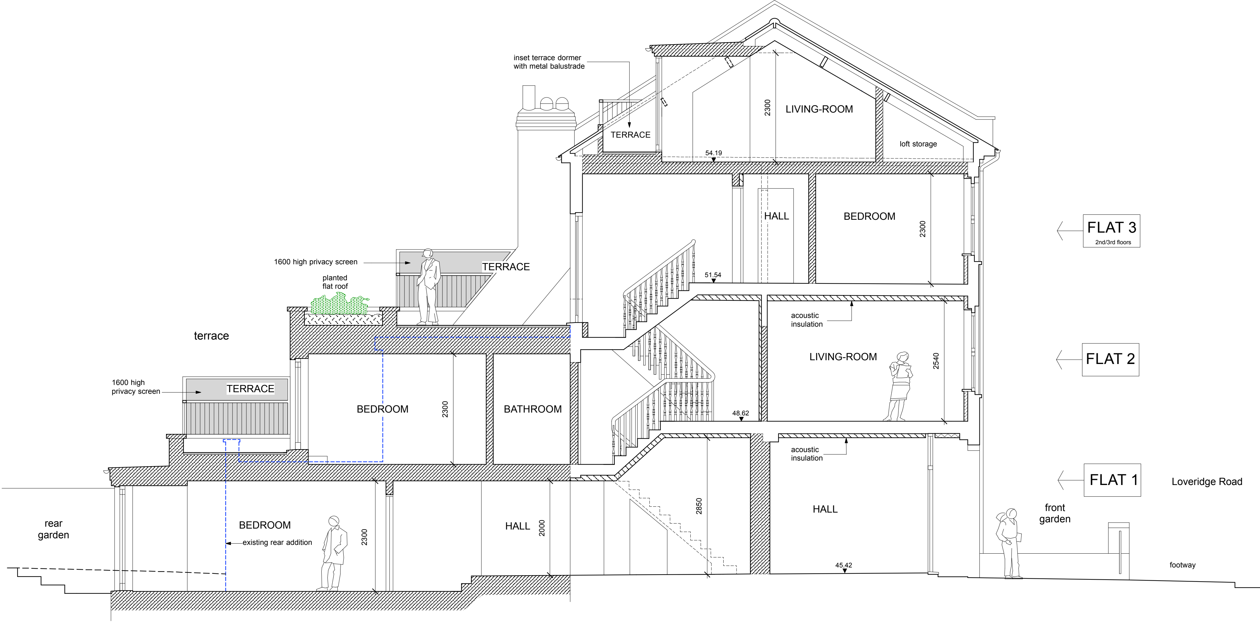
SECTION A-A
