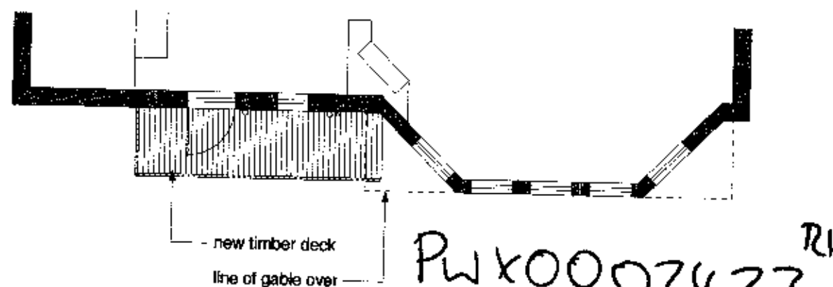
PLAN 1:100
