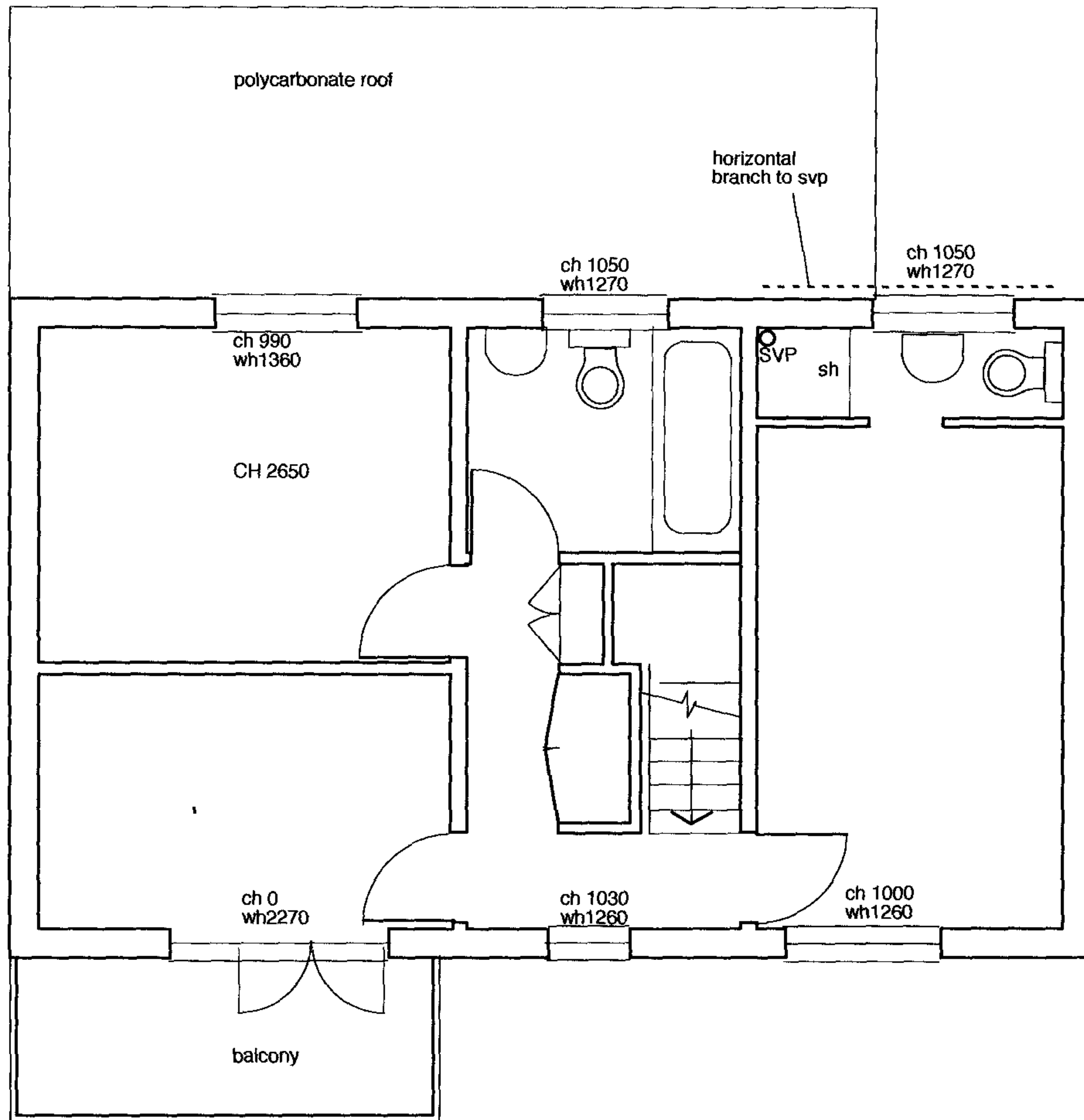
IST FLOOR SURVEY
