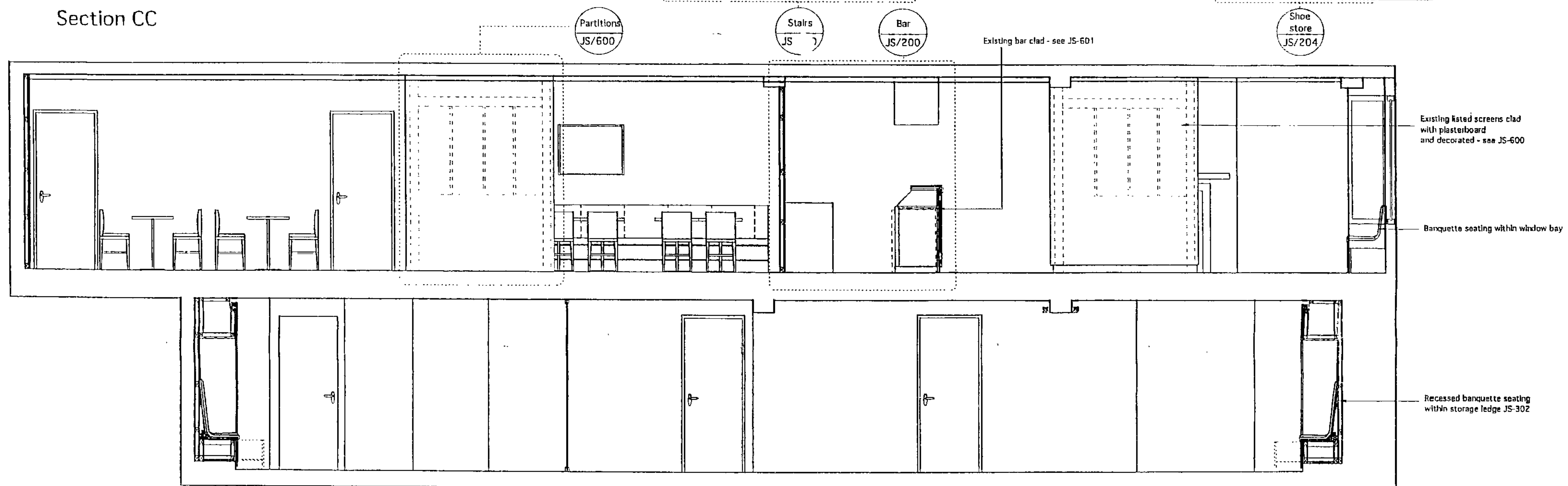
Section DD
