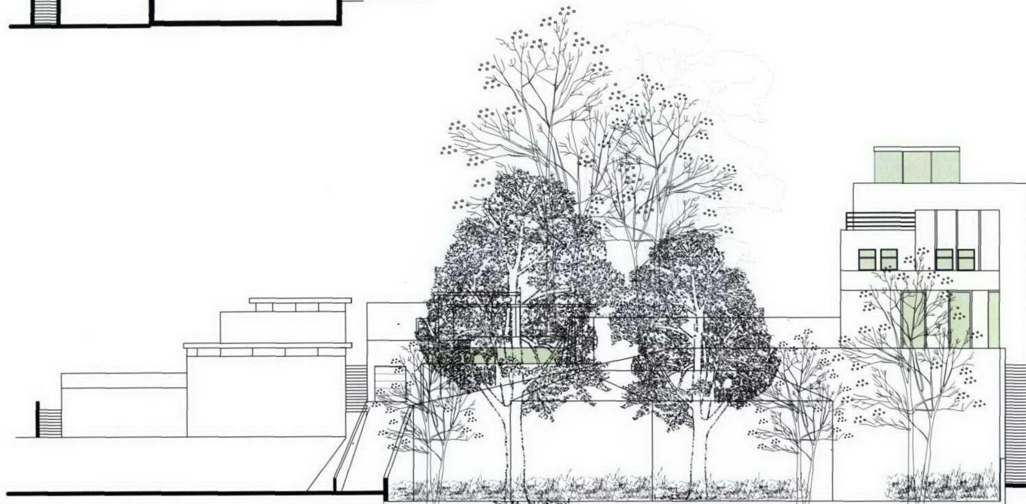
SECTION AA DATUM 0.00
