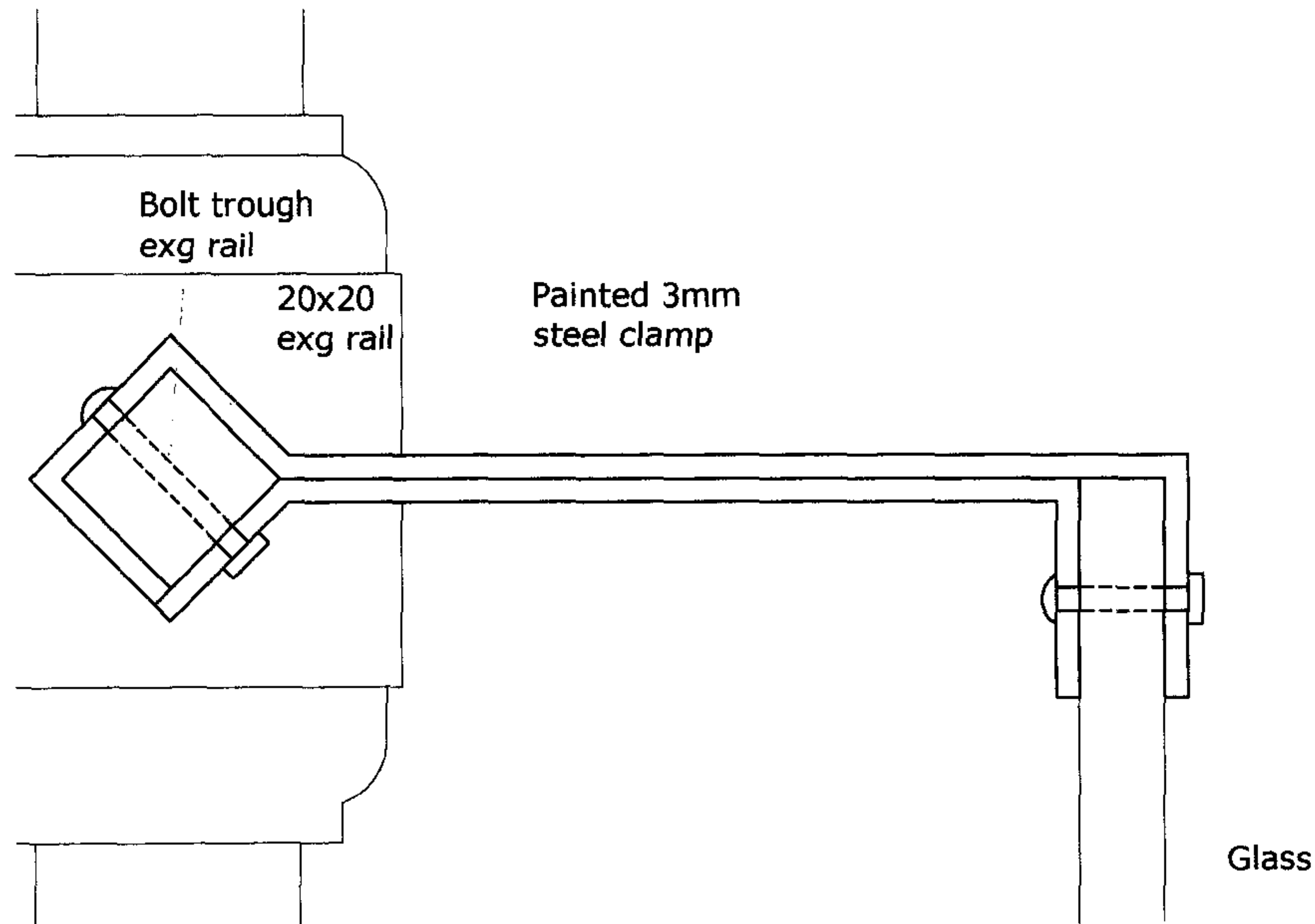
Hinge detail scale 1:1
