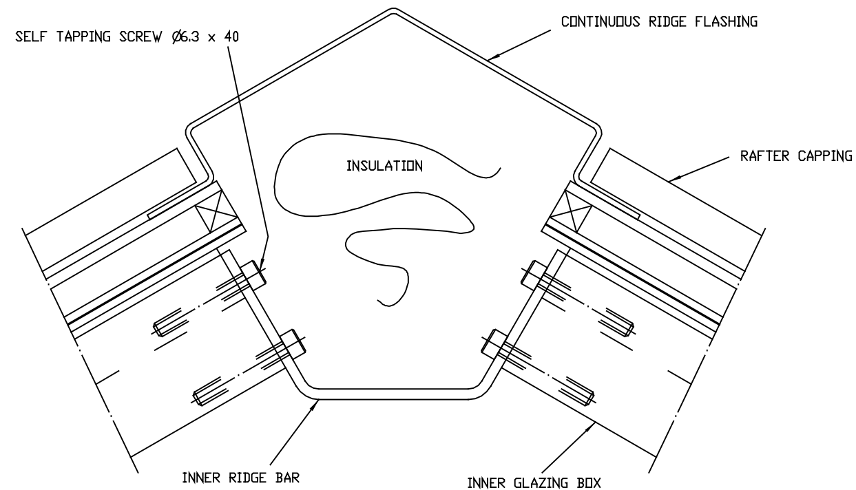
SECTION D-D
