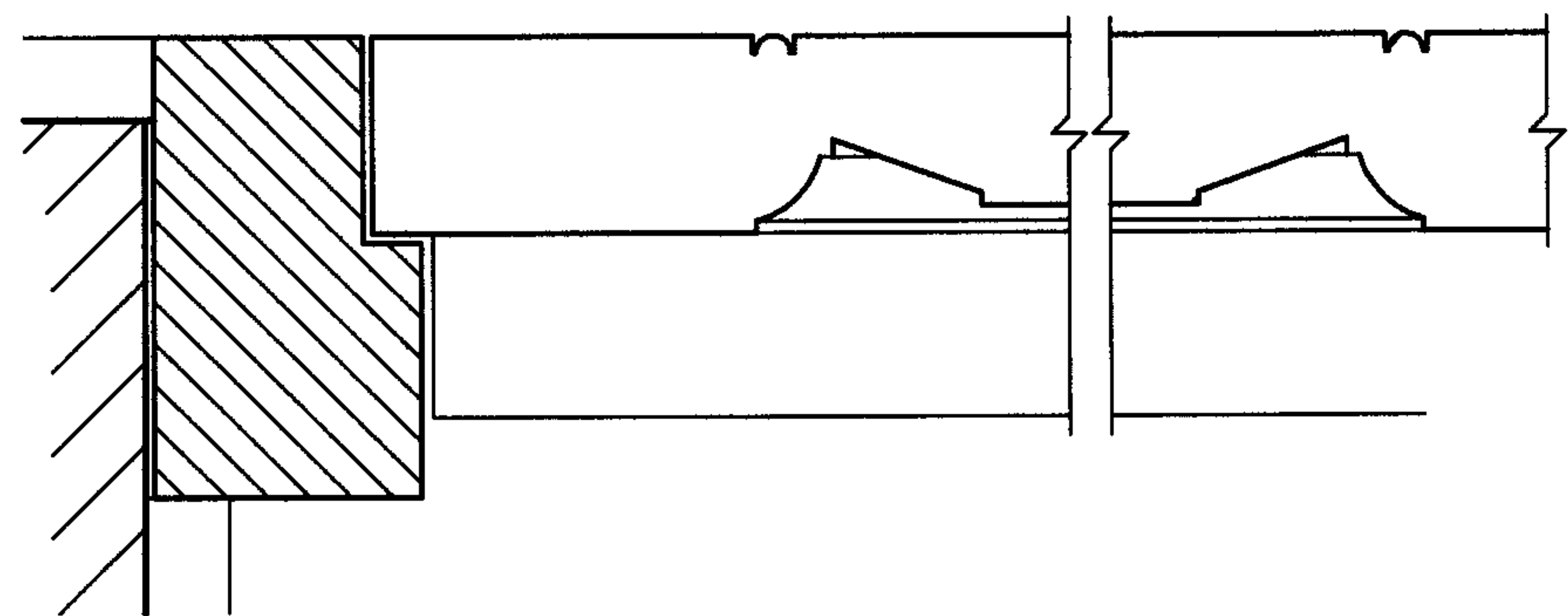
PLAN: DOOR JAMB
