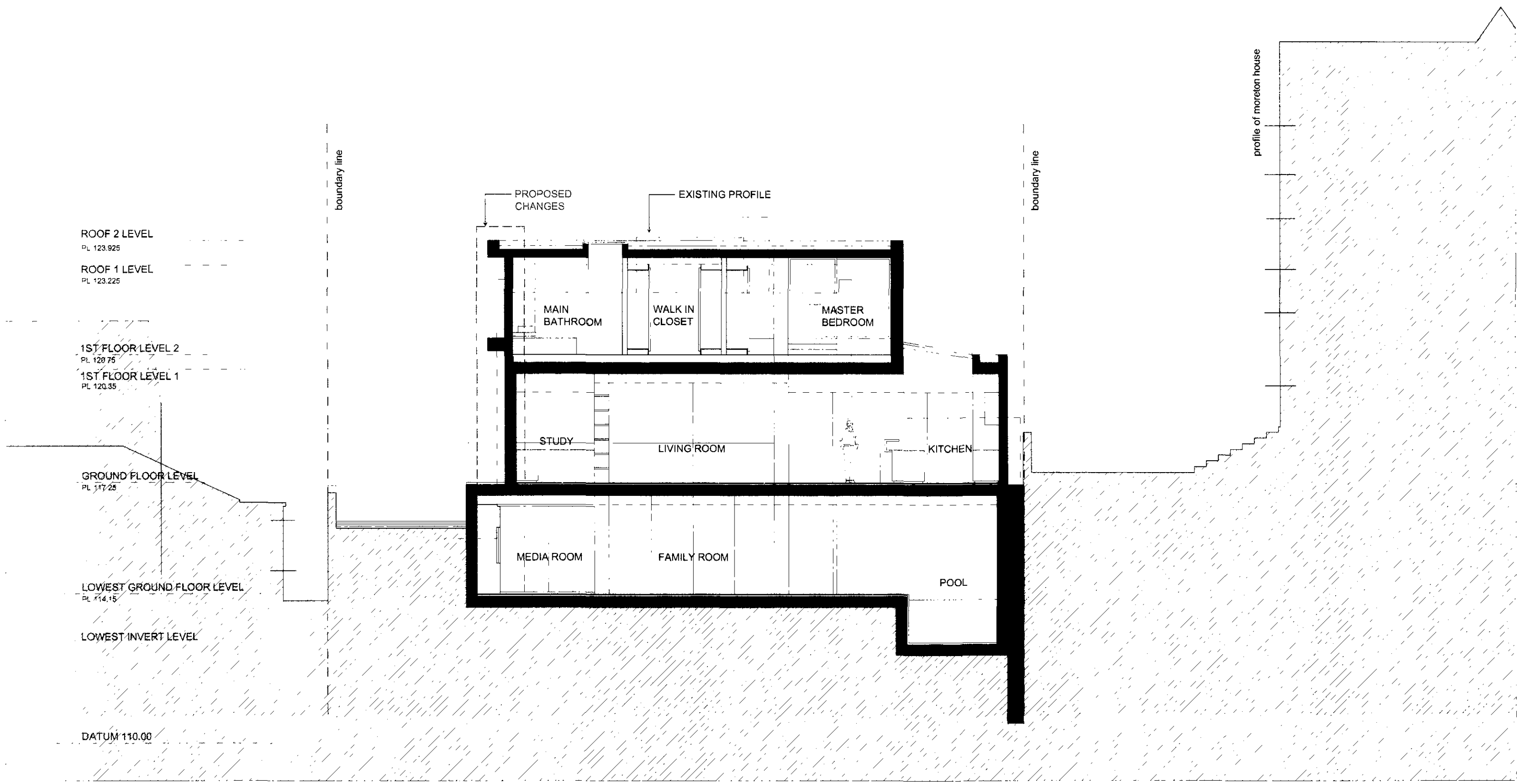
SECTION A-A
