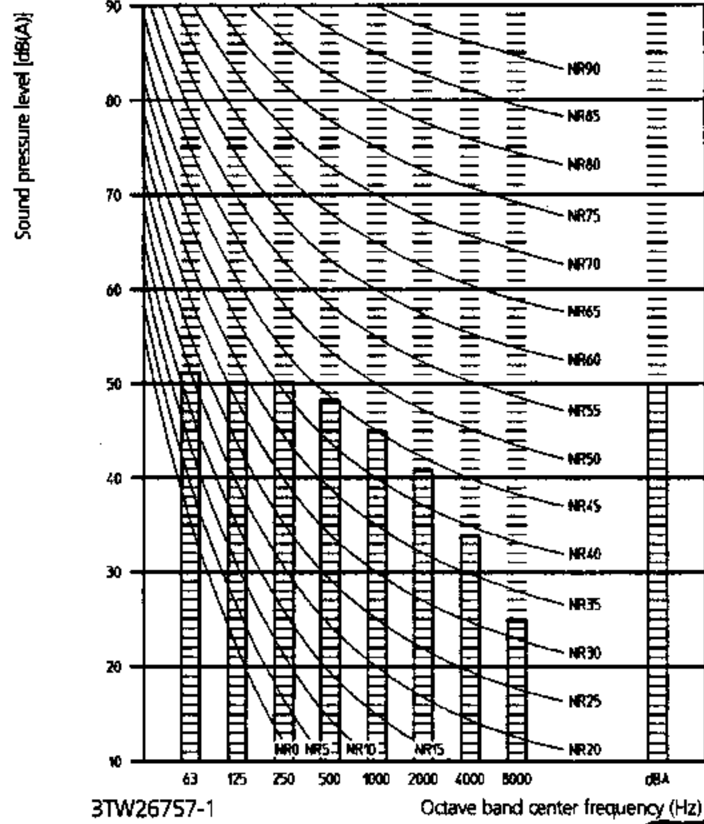
RZQ125B8V3B - Cooling RZQ125B7W1B
