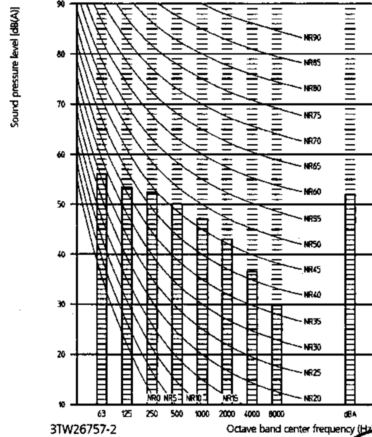
RZQ125B8V3B - Heating RZQ125B7W1B
