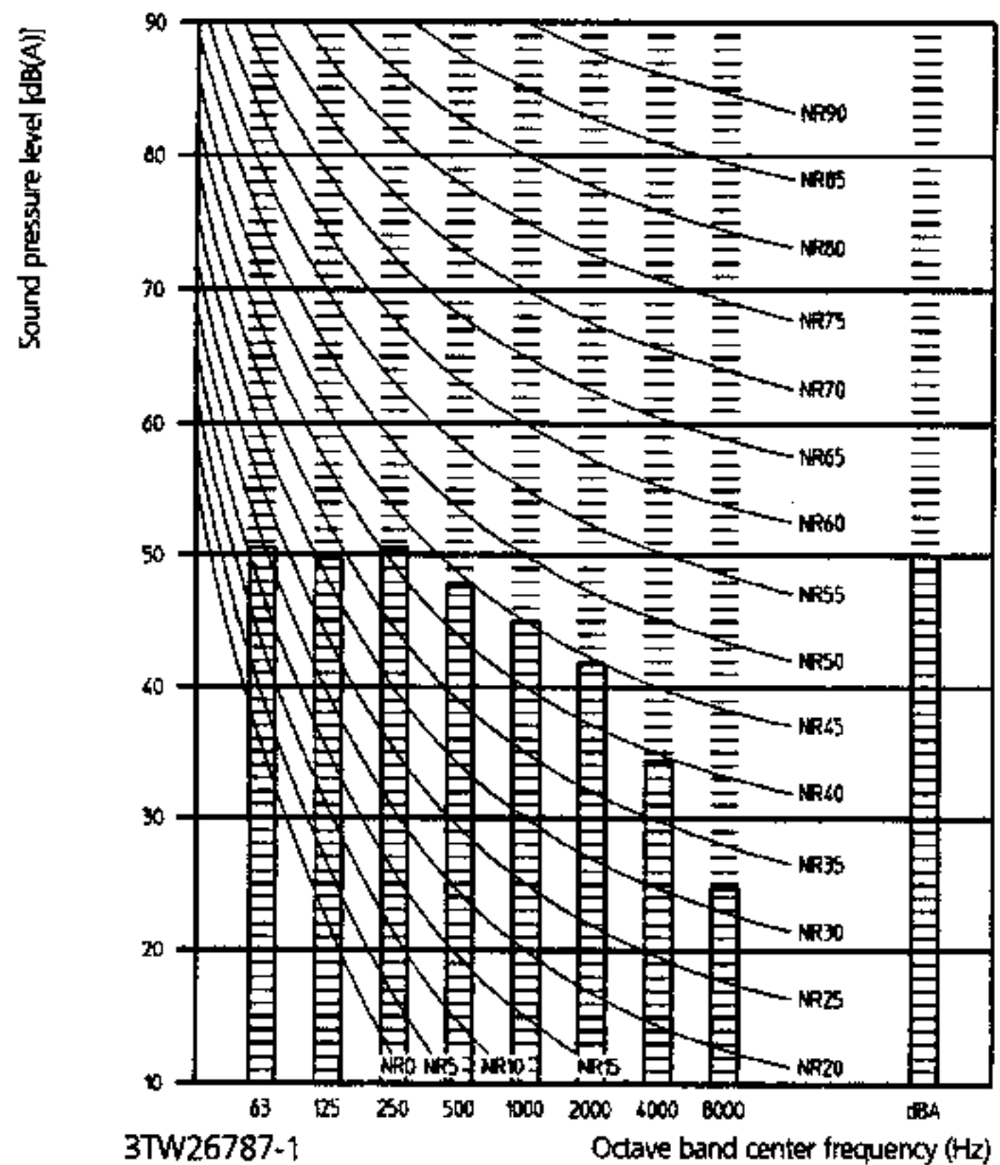
RZQ140B8V3B - Cooling
