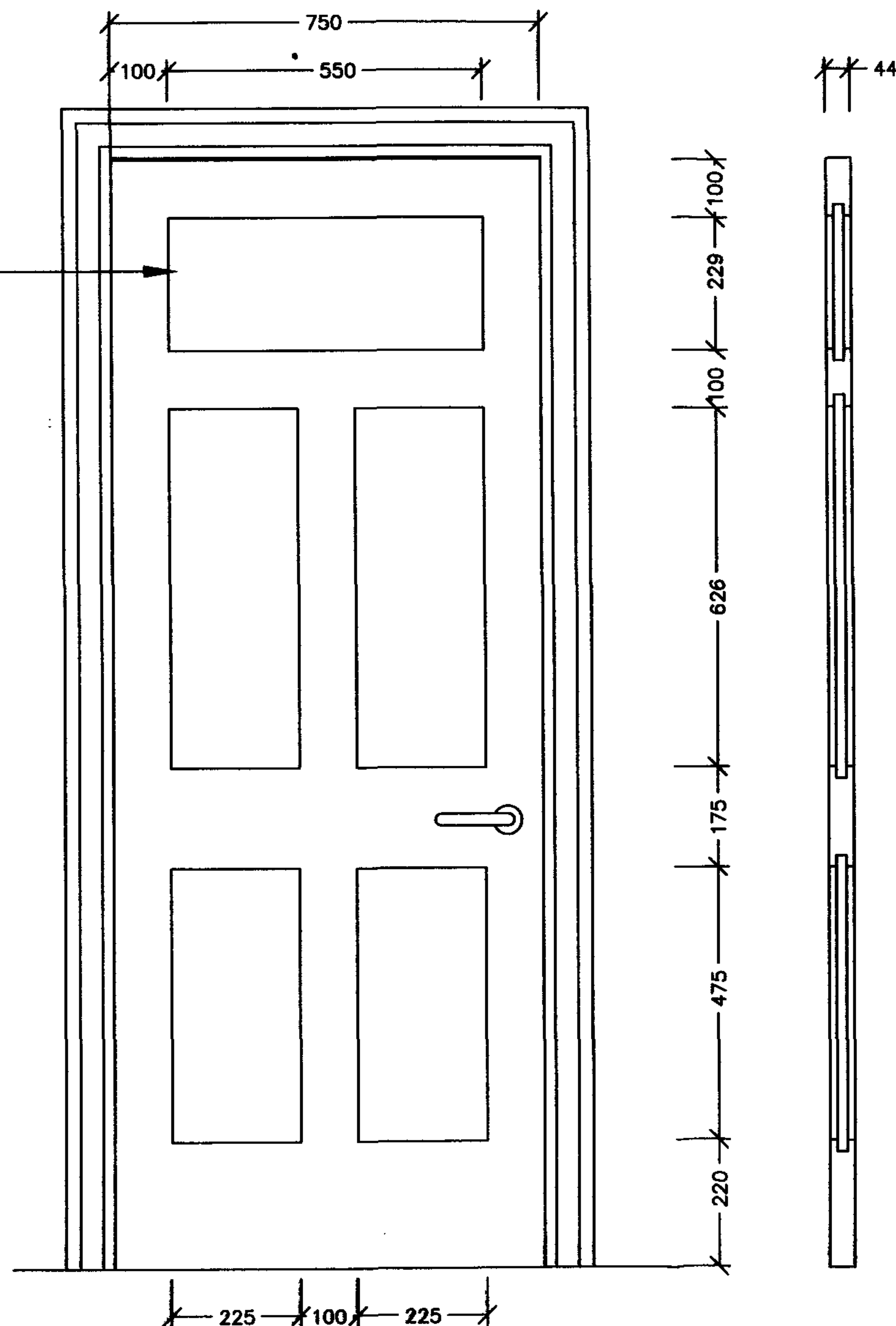
Plan ~ 1:5
