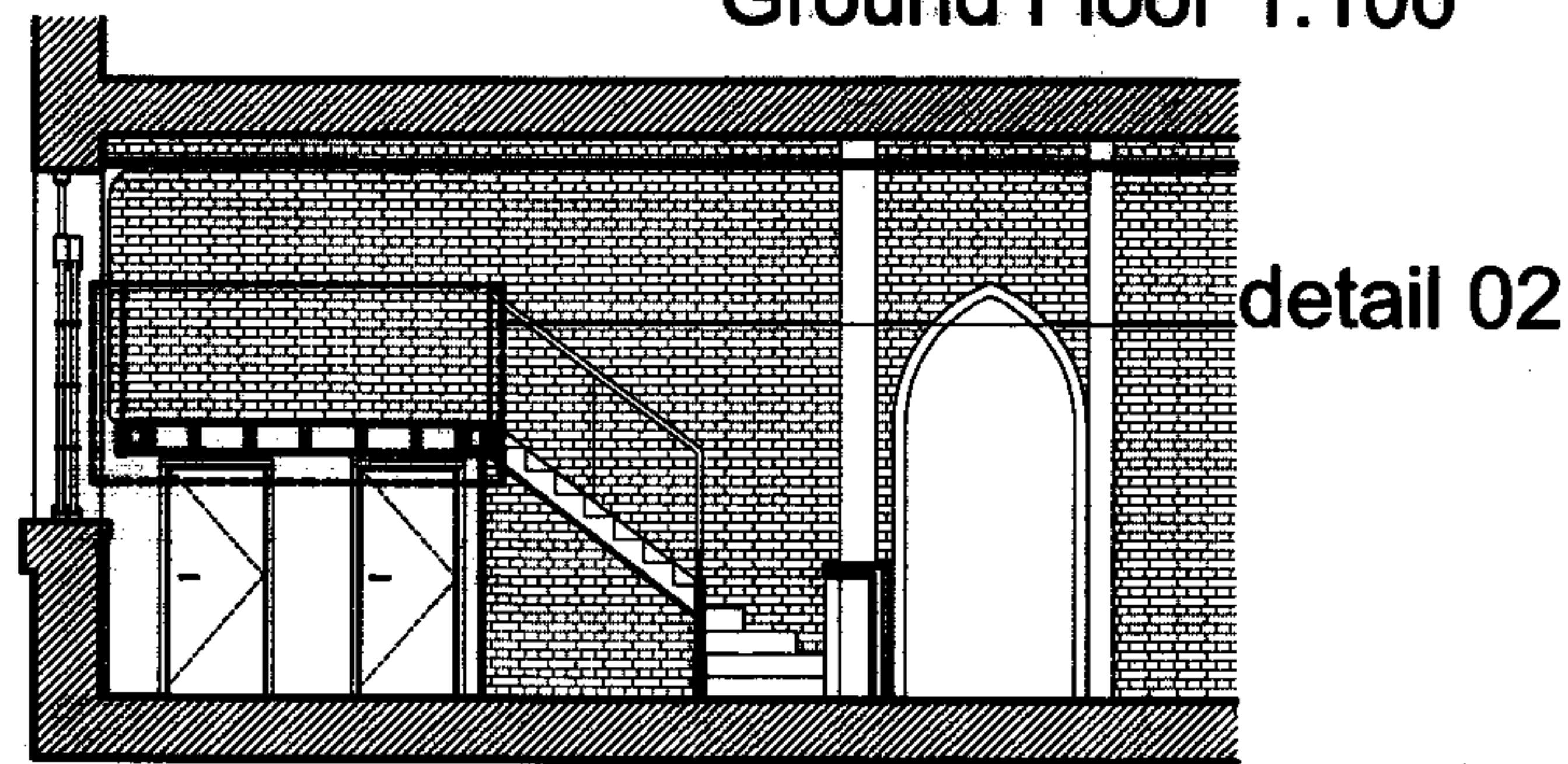
Section A-A 1:100
