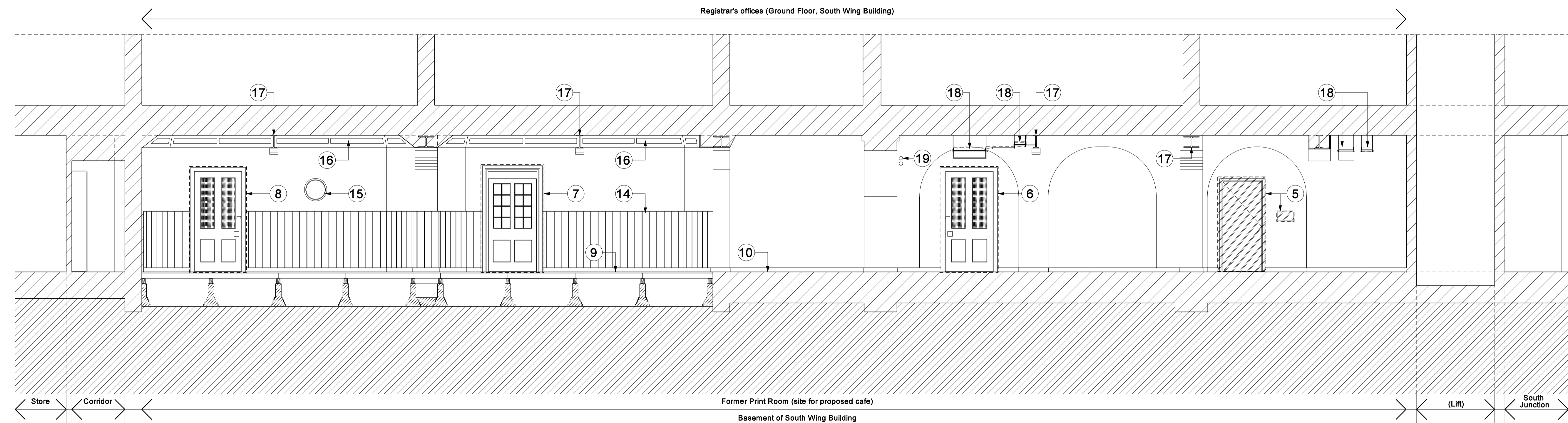
Section DD - Existing
