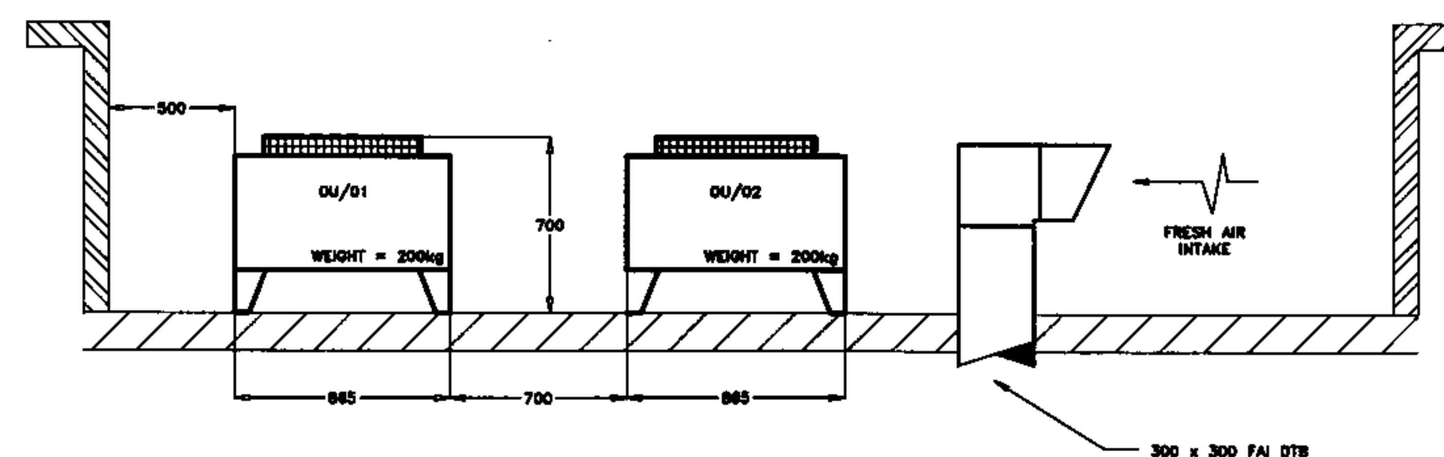
ELEVATION A-A
