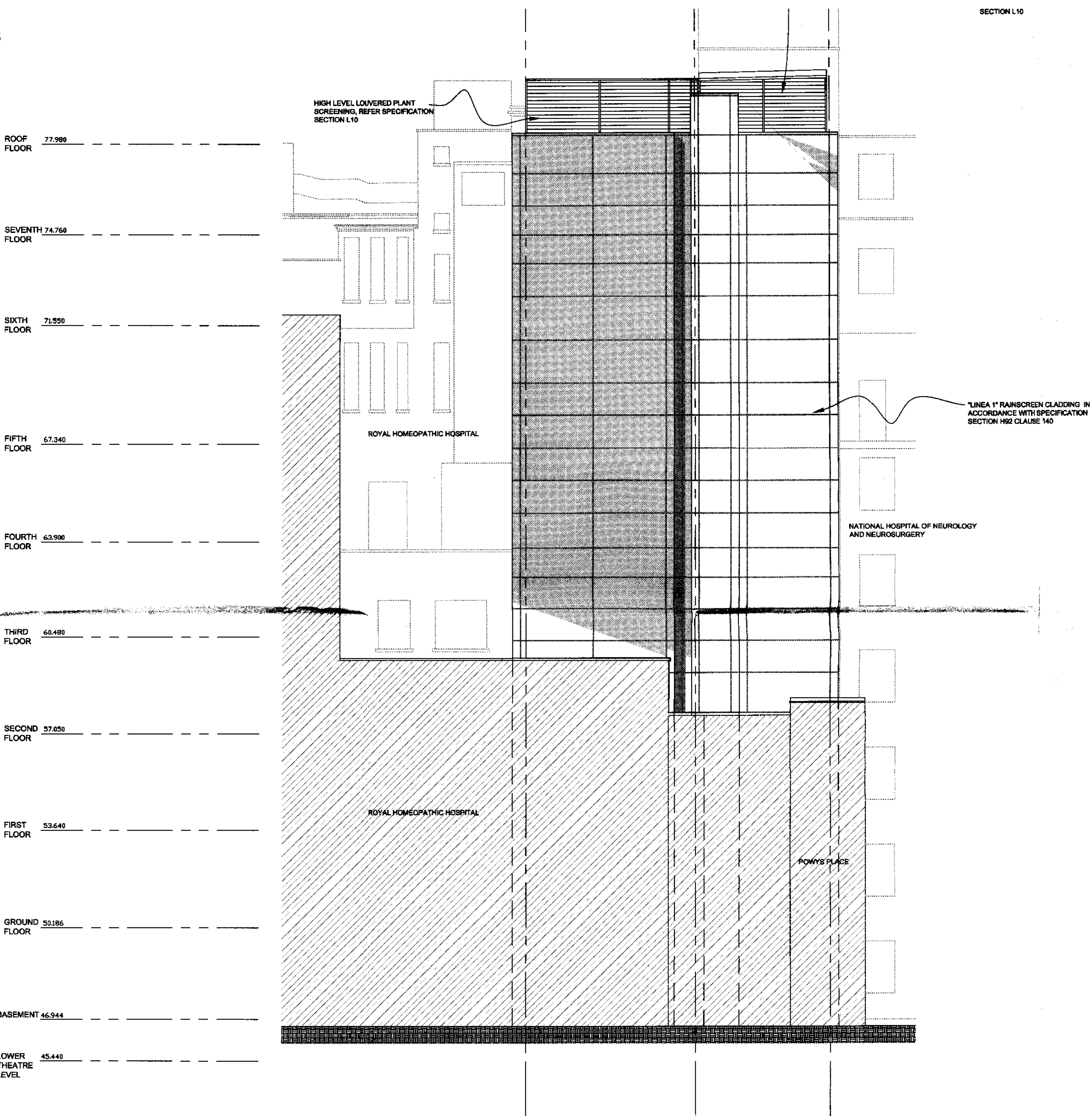
Elevation 3
