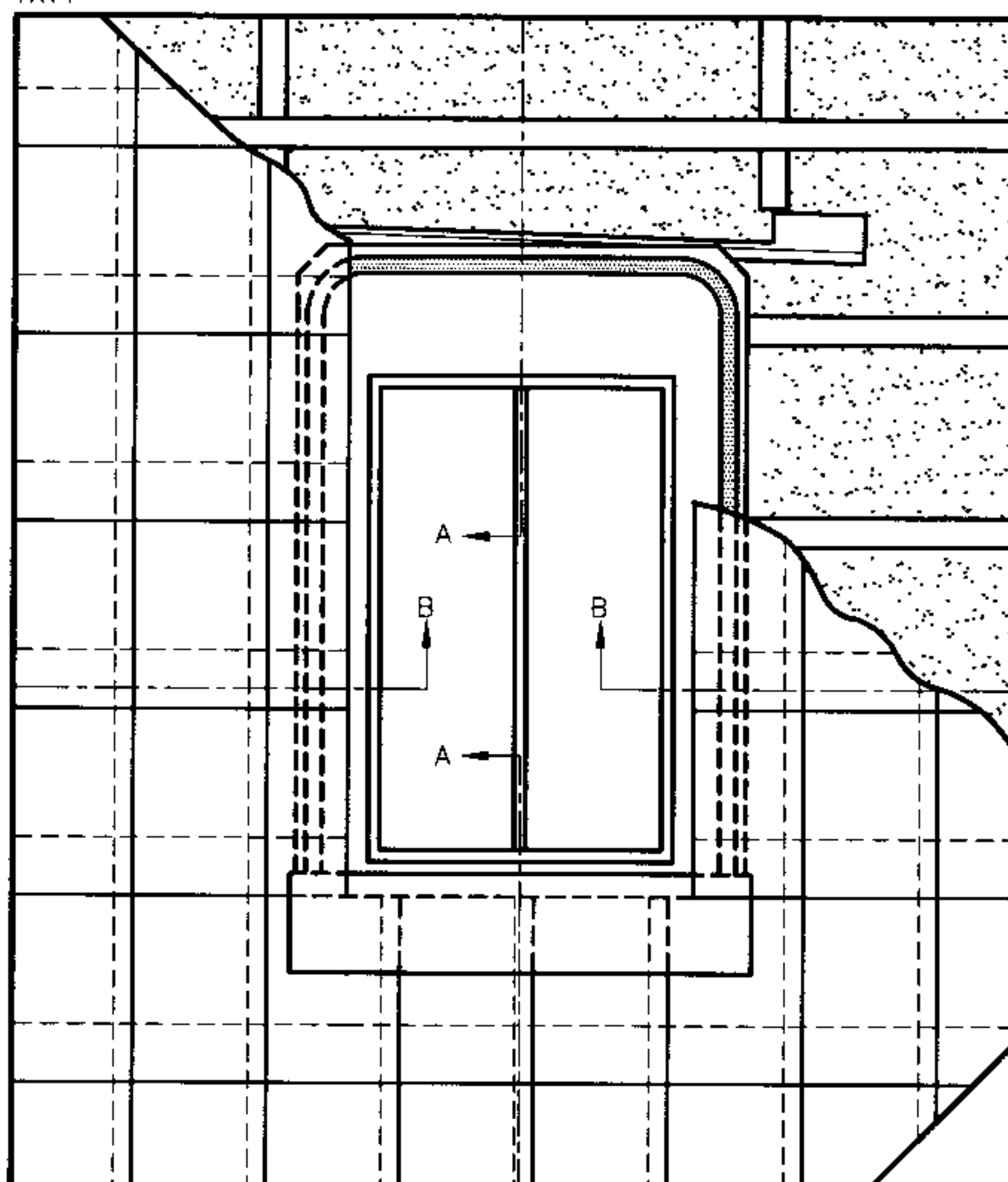
1:20 ELEVATION
