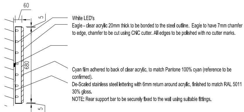
Section A-A 1:20
