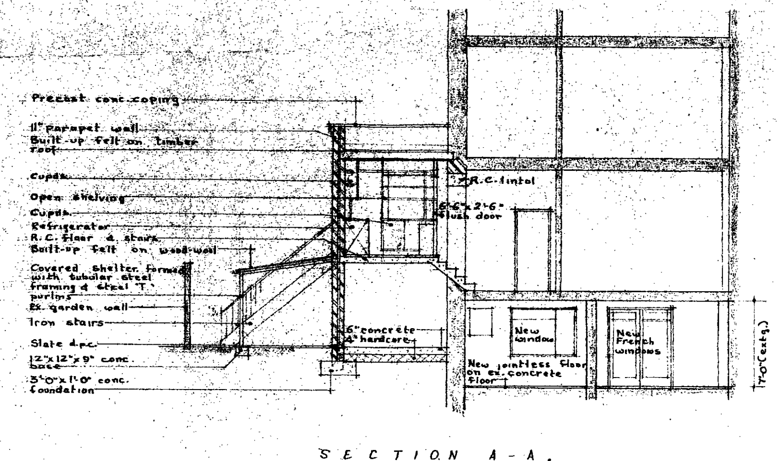
SECTION A-A.
