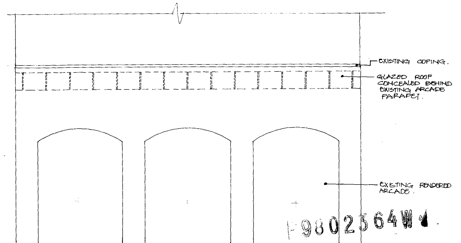
ELEVATION
