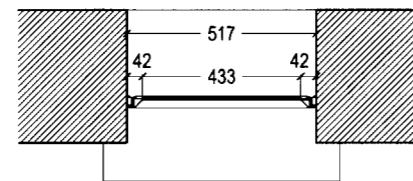
Existing Jamb
