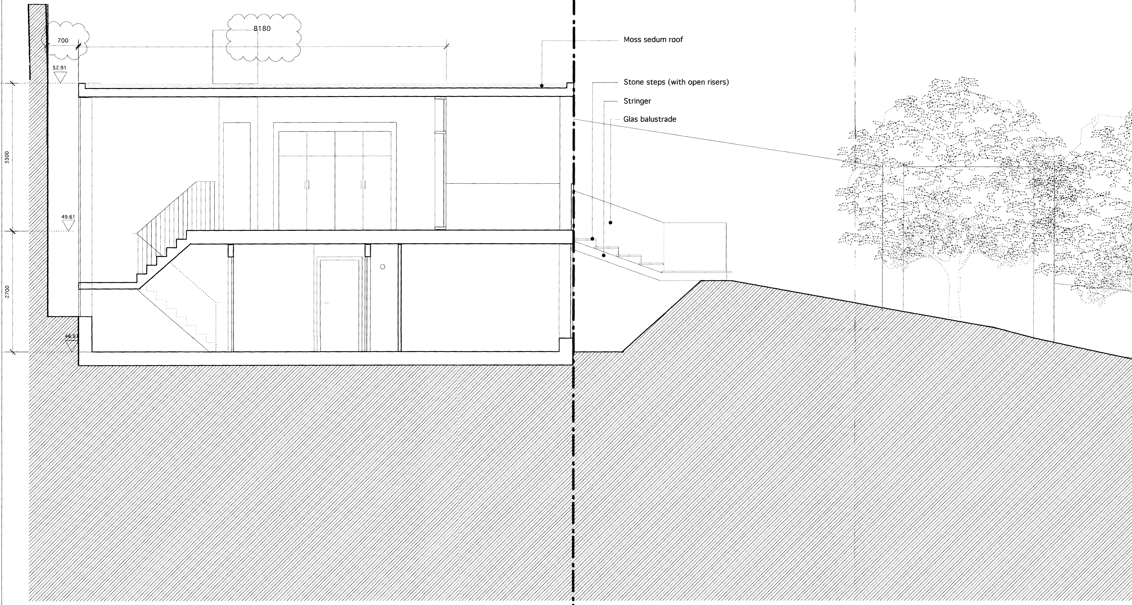
Section A-A
