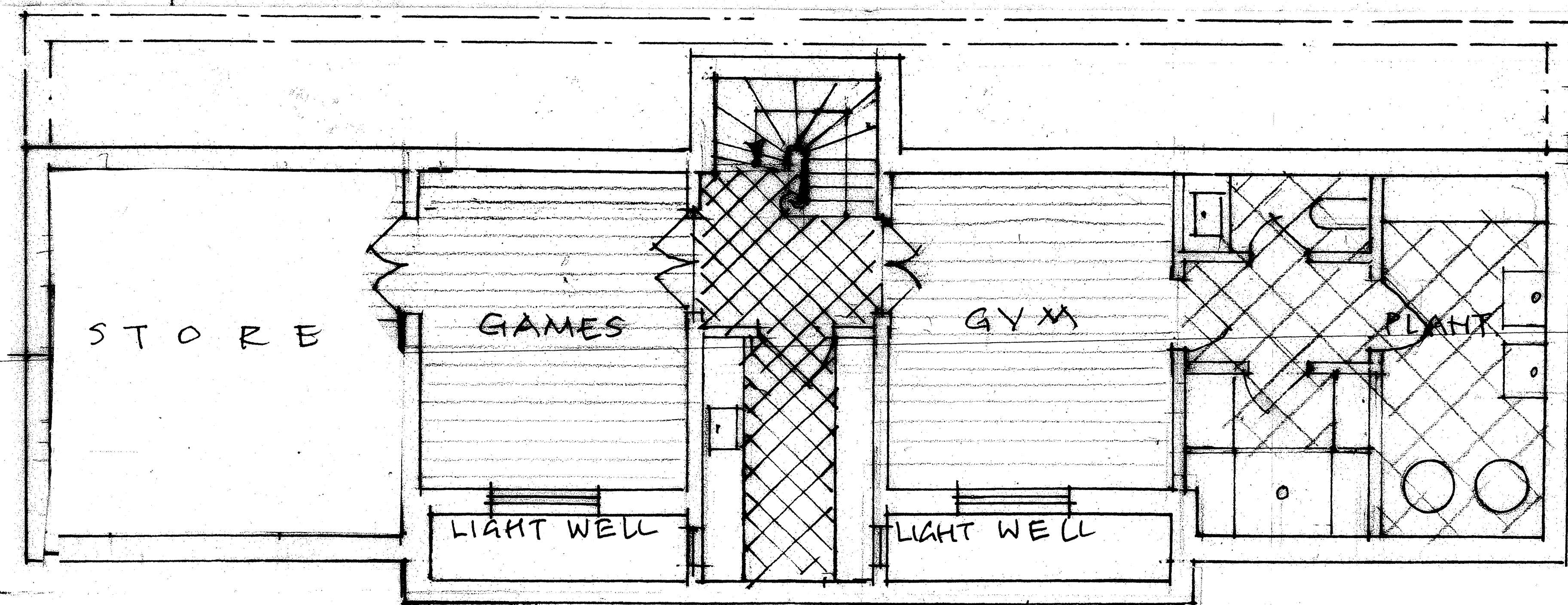
BASEMENT 1:50
