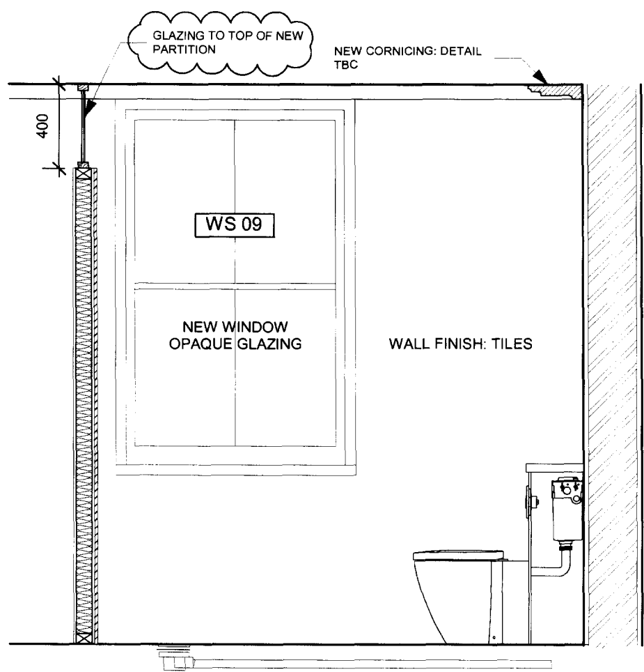
ELEVATION A
