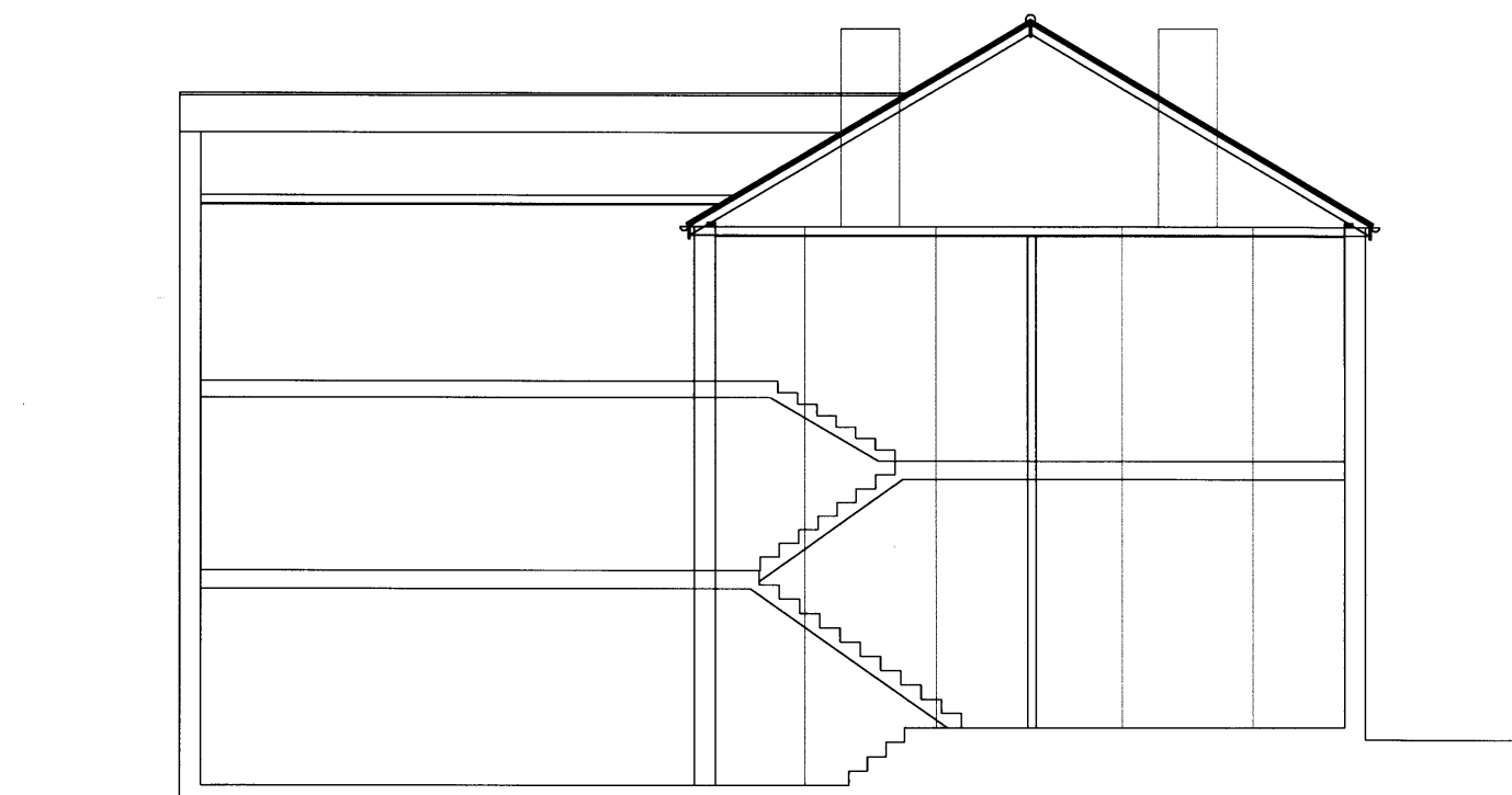
SECTION A-A
