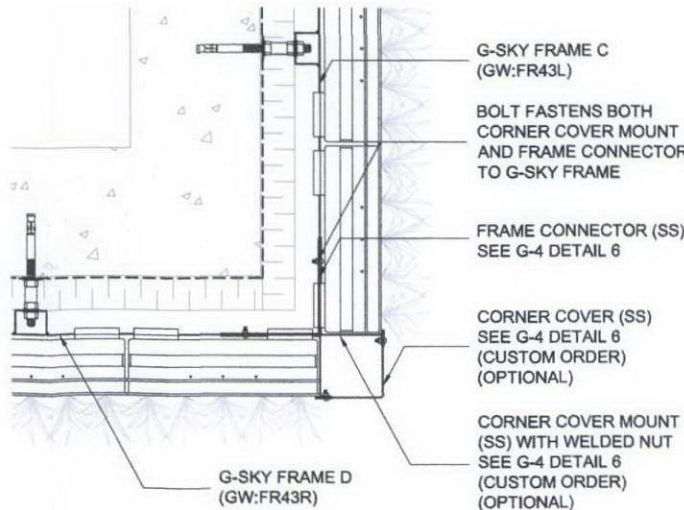
CORNER DETAIL (EIFS SYSTEM)
