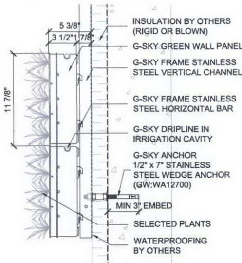
SIDE VIEW (EIFS SYSTEM)
