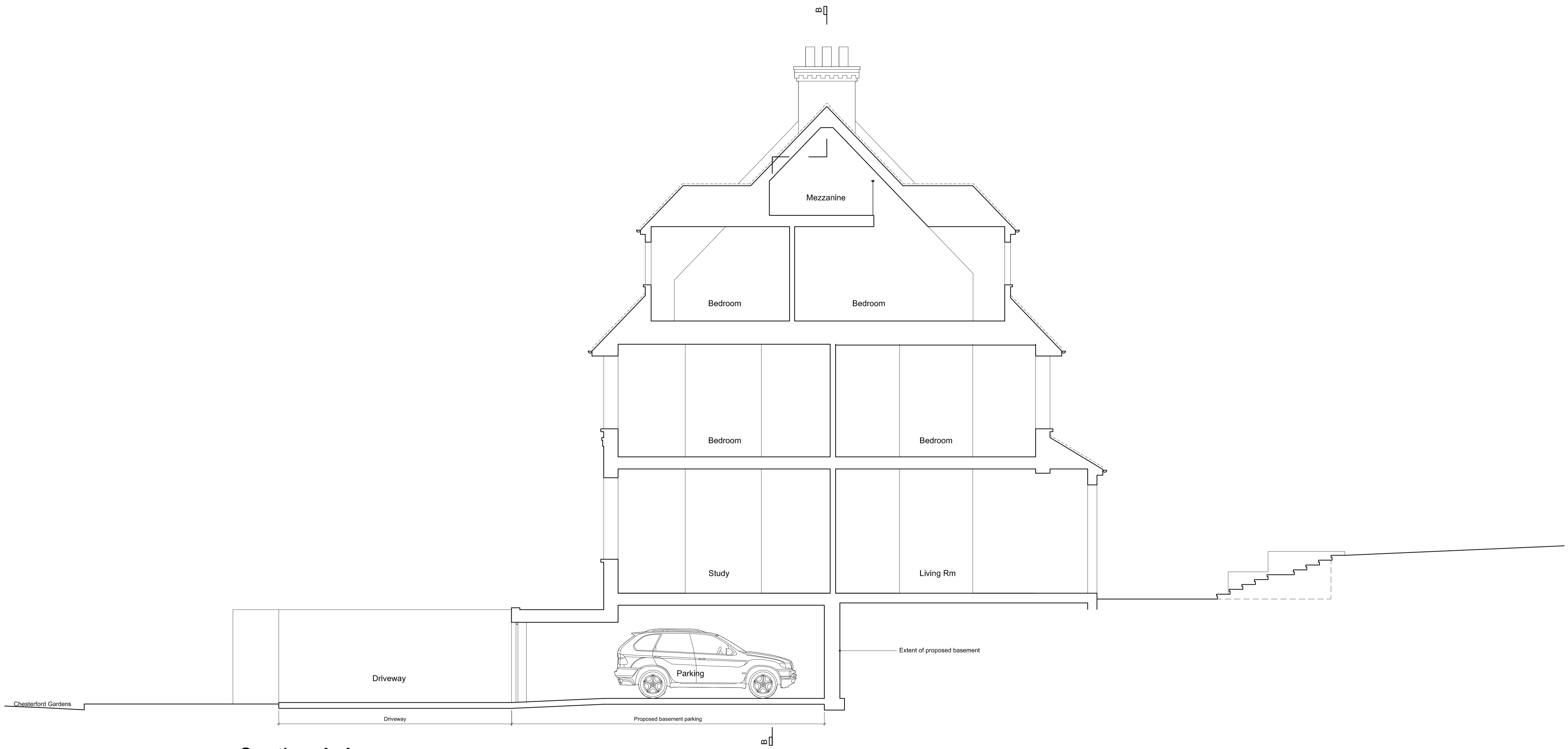
Section A-A 1:50
