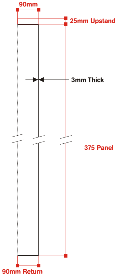
Fascia Side Section Scale: 1:10@A3
