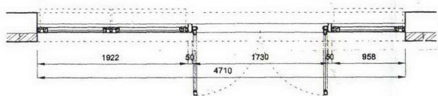
PLAN 1:50
