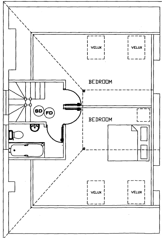
LOFT PLAN
