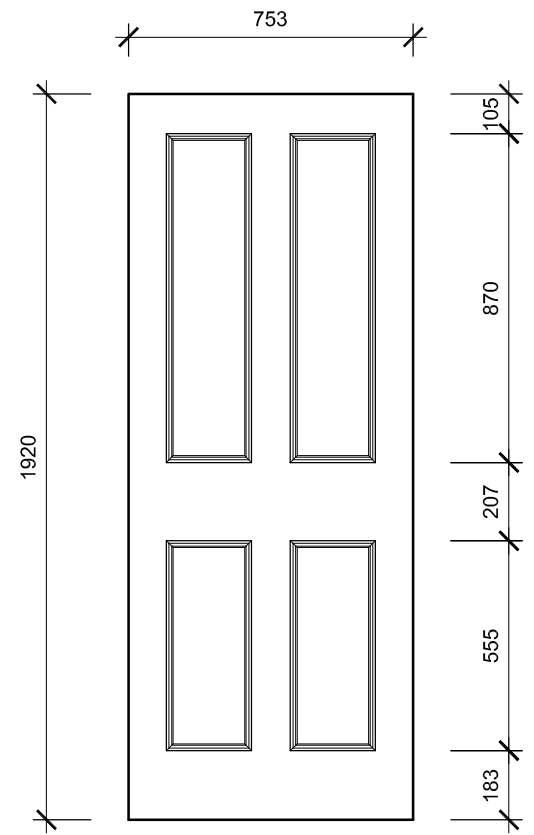
9. Existing Door Type J Scale 1:20
