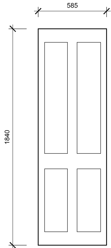
12. Existing Door Type M Scale 1:20
