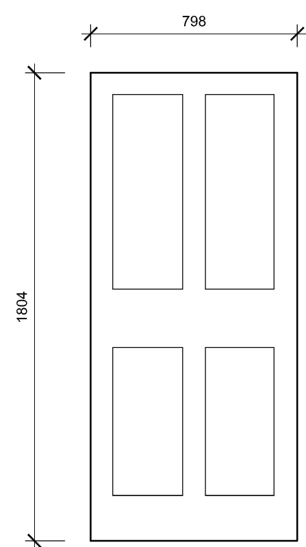
13. Existing Door Type N Scale 1:20
