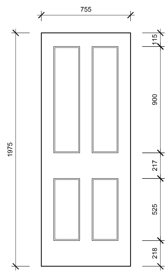
8. Existing Door Type H Scale 1:20
