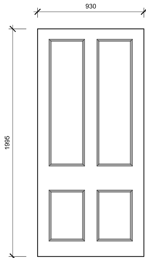
11. Existing Door Type L Scale 1:20
