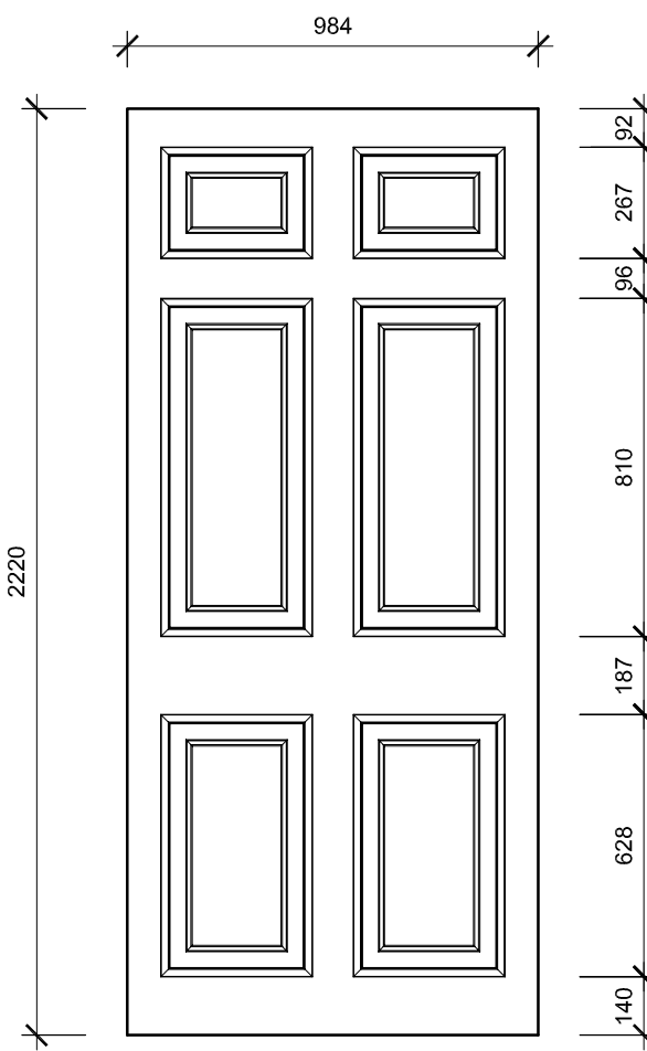
4. Existing Door Type D Scale 1:20
