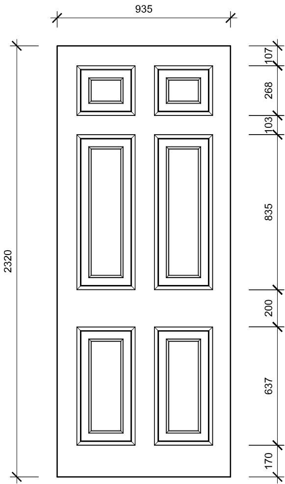
2. Existing Door Type B Scale 1:20
