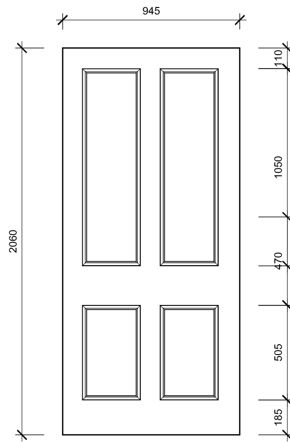
5. Existing Door Type E Scale 1:20
