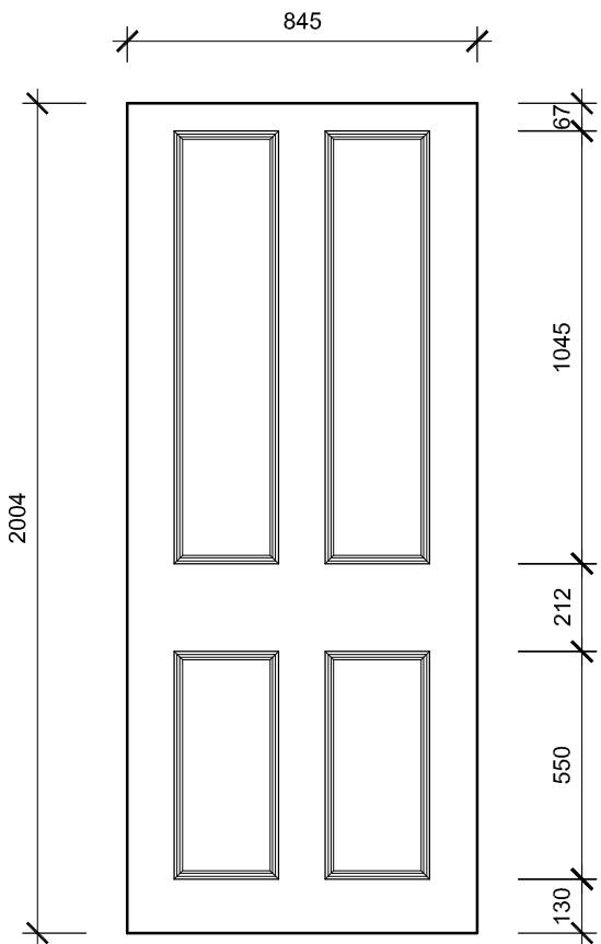
7. Existing Door Type G Scale 1:20
