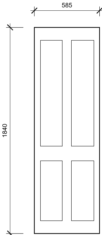
12. Existing Door Type M Scale 1:20
