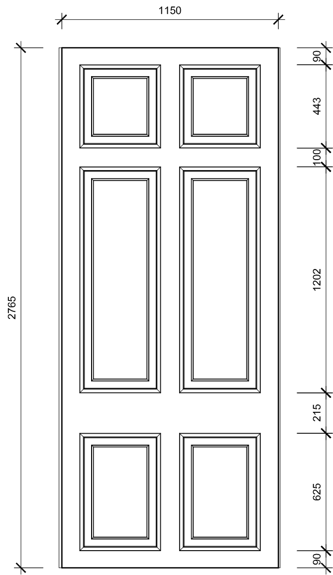
1. Existing Door Type A Scale 1:20
