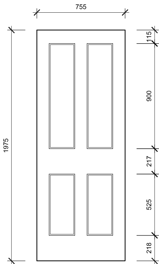
8. Existing Door Type H Scale 1:20
