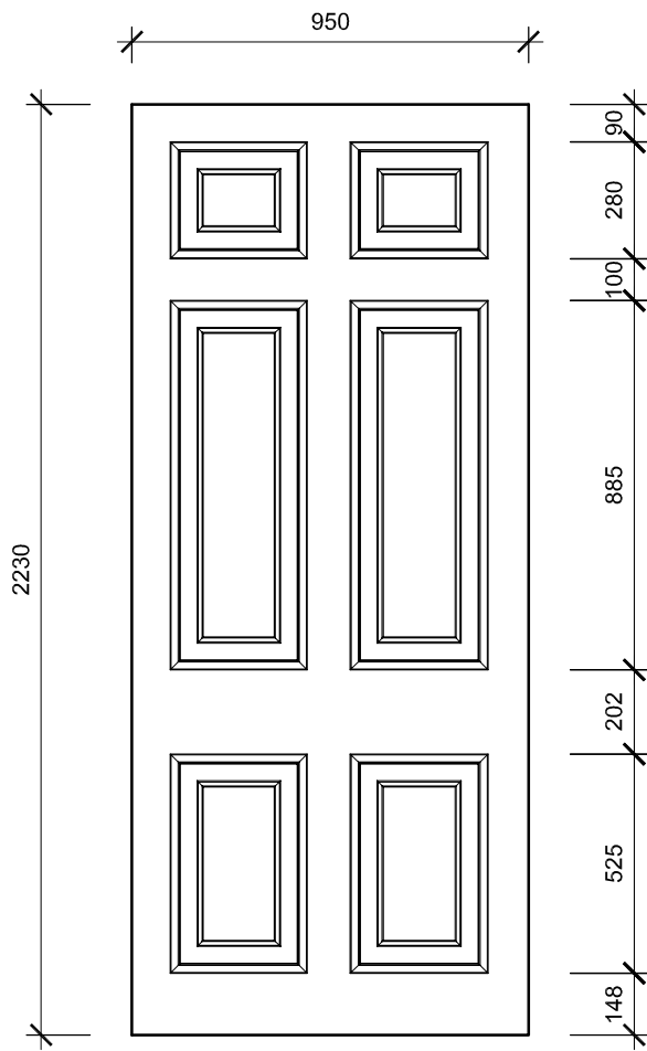
3. Existing Door Type C Scale 1:20
