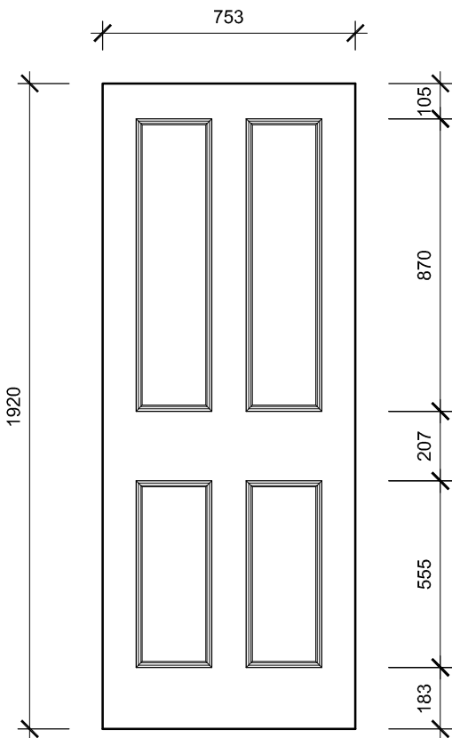
9. Existing Door Type J Scale 1:20
