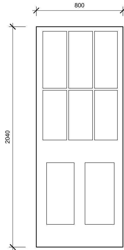
10. Existing Door Type K Scale 1:20
