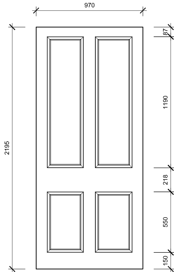
6. Existing Door Type F Scale 1:20
