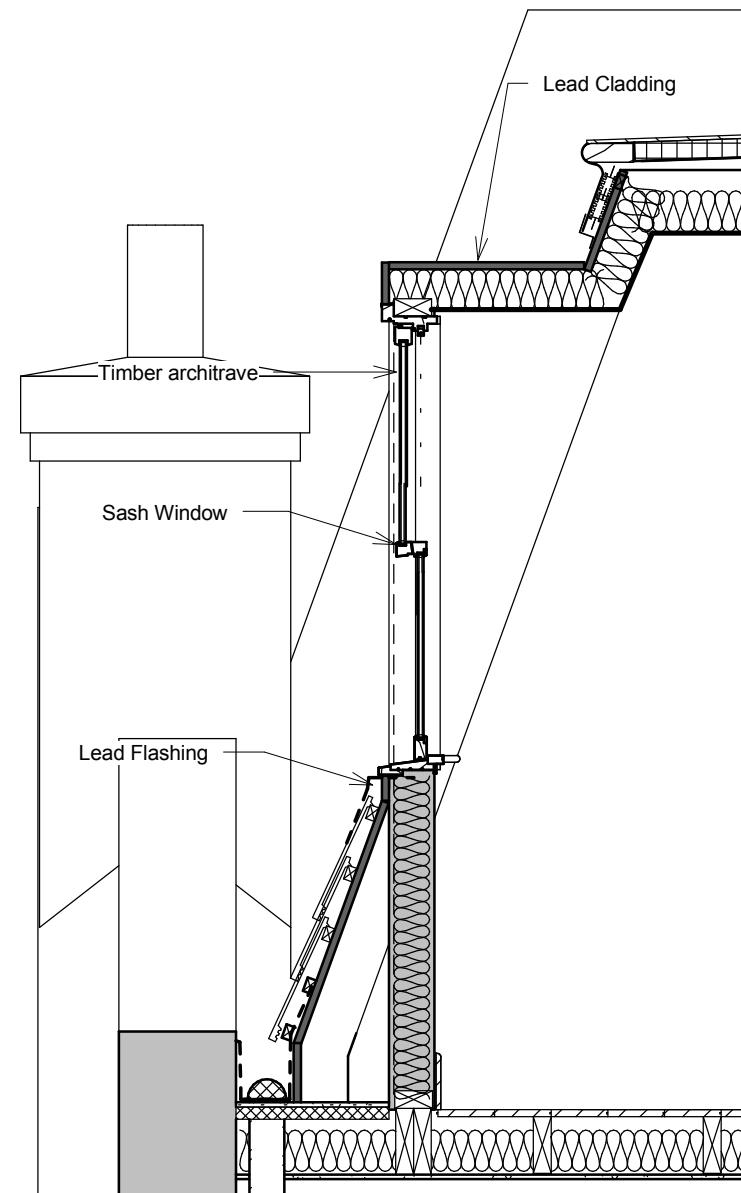
1 Dormer Section 1 : 20
