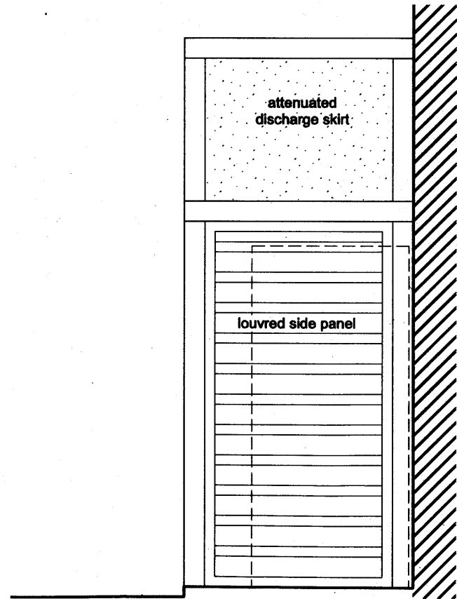
ELEVATION B 1:25
