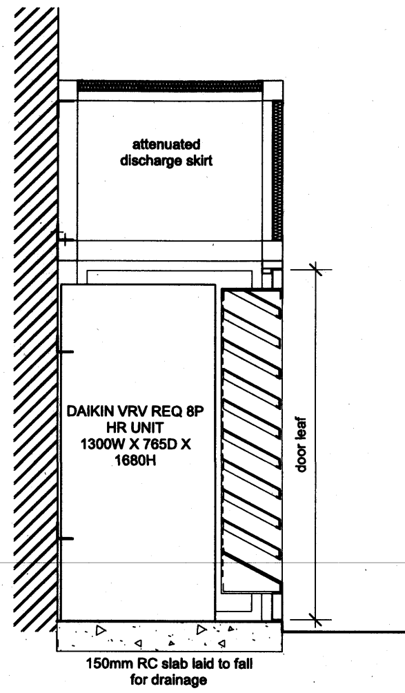
SECTION 1:25
